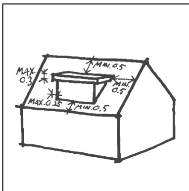
Plaatsing dakkapel.
