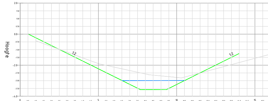
Dwarsprofiel 5
