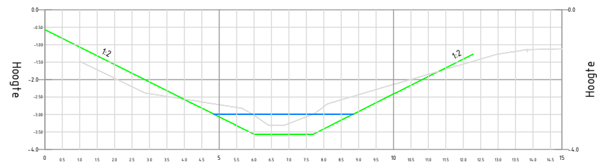
Dwarsprofiel 2
