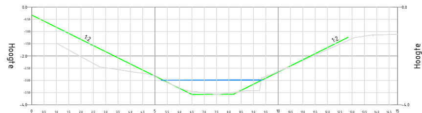
Dwarsprofiel 1
