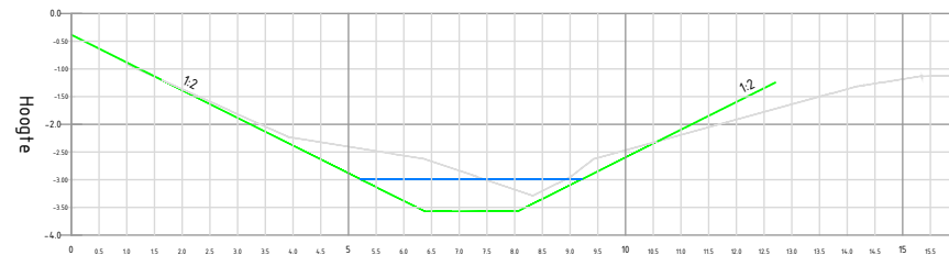
Dwarsprofiel 4
