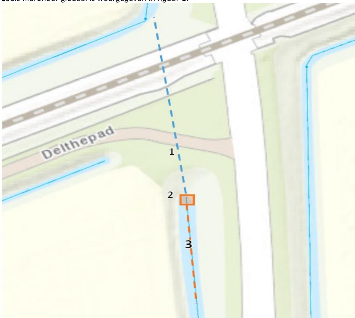
Figuur 1: Bestaande spoorduiker aangegeven met 1, benodigde inspectieput aangegeven met 2, te leggen duiker aangegeven met 3.
