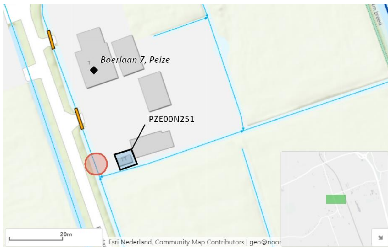
Figuur 1: Situatietekening met gewenste locatie van de te leggen dam met duiker (rode cirkel)
