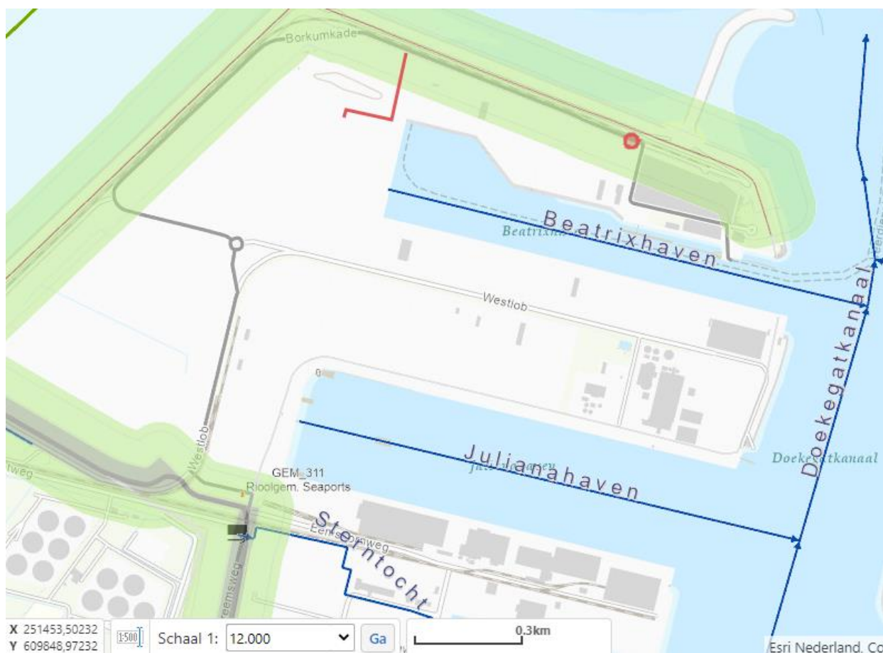
Figuur 1: Schematische tekening van de werkzaamheden. De rode lijn geeft het aan te leggen glasvezeltracé weer, de rode cirkel geeft de locatie weer van de werkzaamheden voor het wijzigen van lasgaten.
