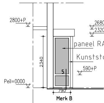
Aanzicht A
