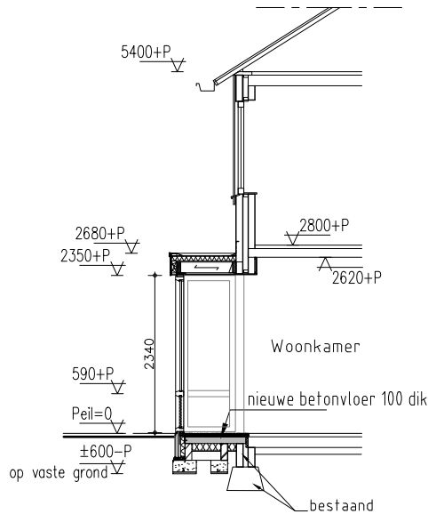
doorsnede nieuw
