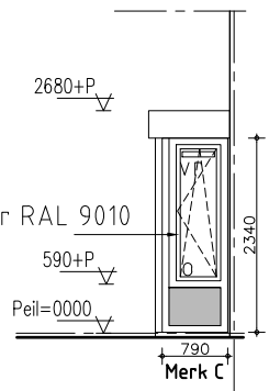
Aanzicht B
