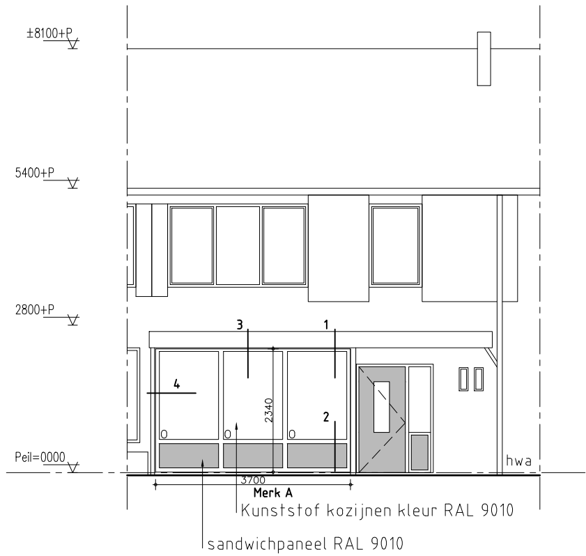
voorgevel nieuw
