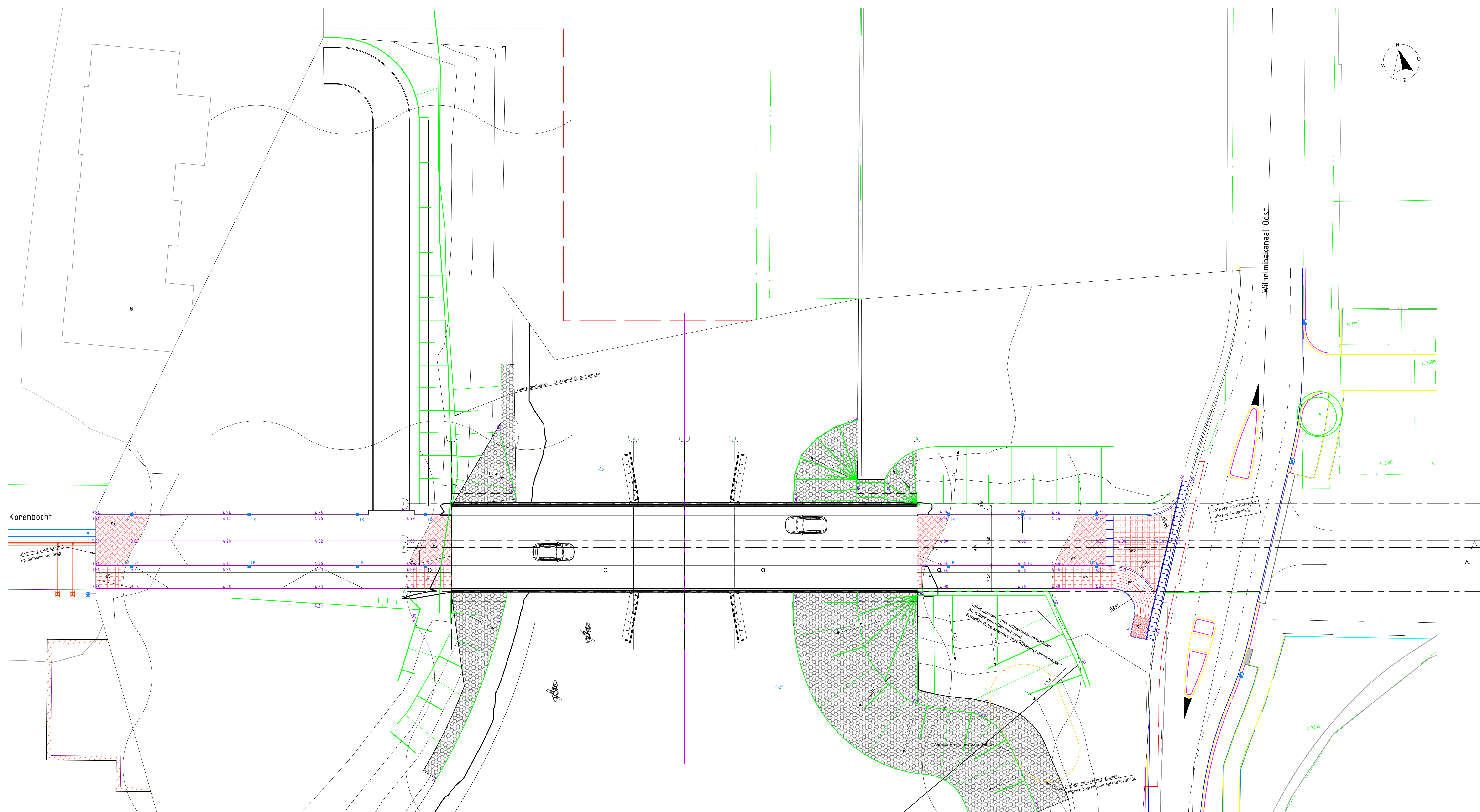
Bovenaanzicht omgeving
