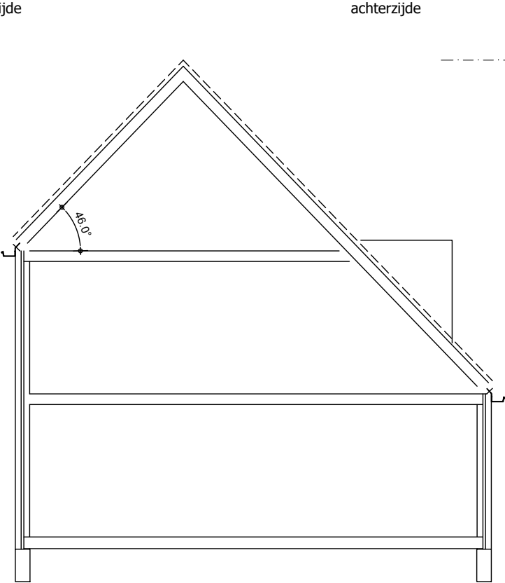
BESTAANDE DOORSNEDE
