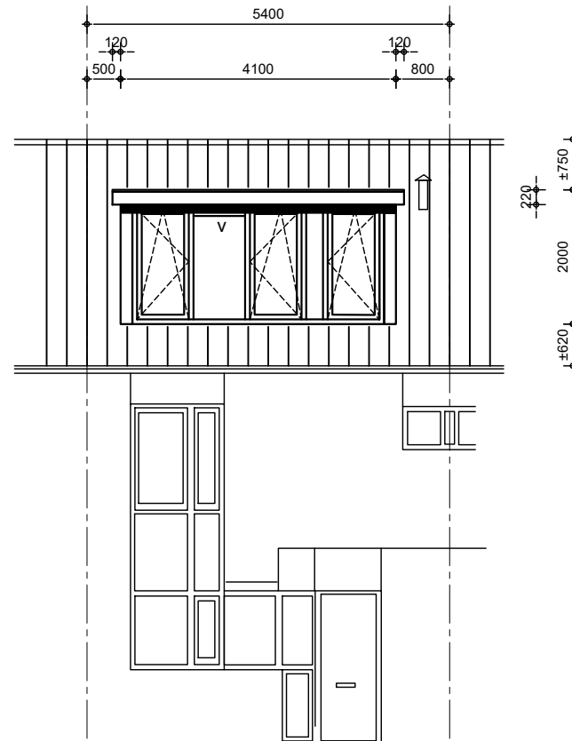
GEWIJZIGDE VOORGEVEL
