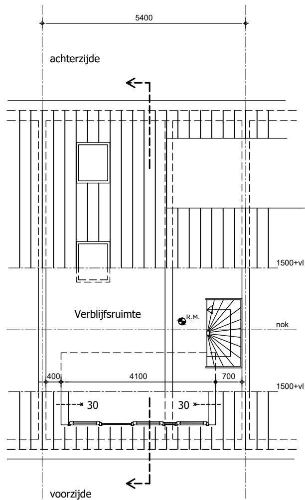
GEWIJZIGDE 2e VERDIEPING
