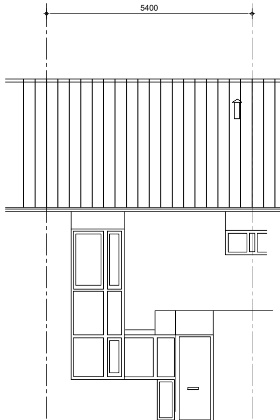
BESTAANDE VOORGEVEL
