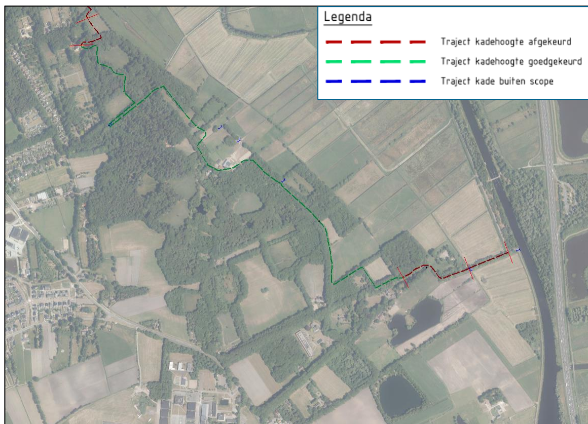
Figuur 1.3: Delen van de kade die versterkt moeten worden (rode lijnen). De groene delen voldoen en blauwe delen liggen buiten de scope van het project.
