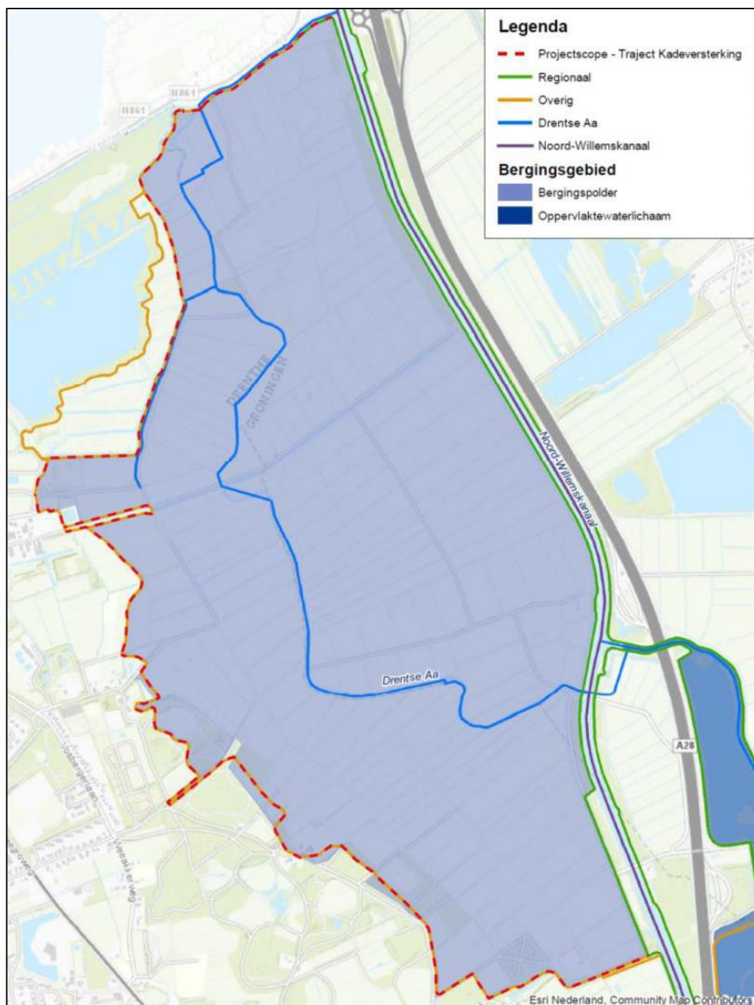
Figuur 1.1: Ligging van de kade. Bron: Waterschap Hunze en Aa's.
