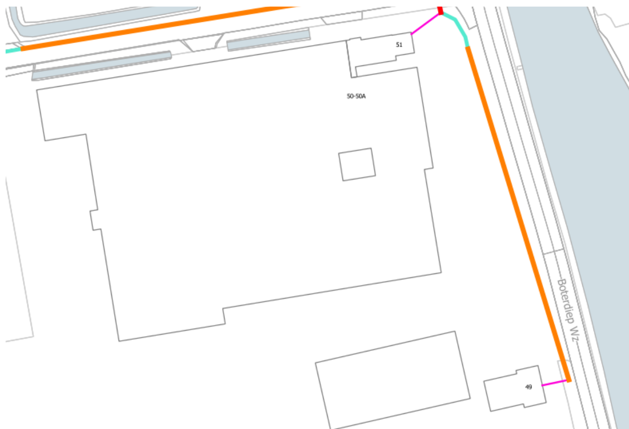
Figuur 2 - Situatietekening locatie gestuurde boring parallel in een regionale waterkering ter hoogte van Boterdiep Westzijde 49 te Bedum (boring weergegeven met oranje streep)
