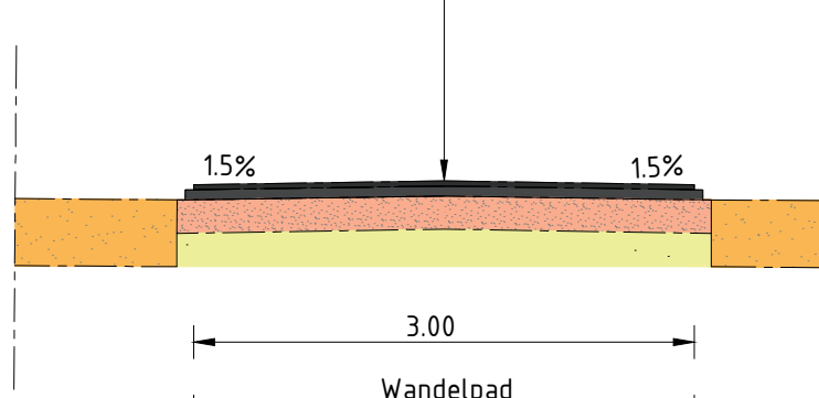
Fietsroute A-A SCHAAL 1 : 50
