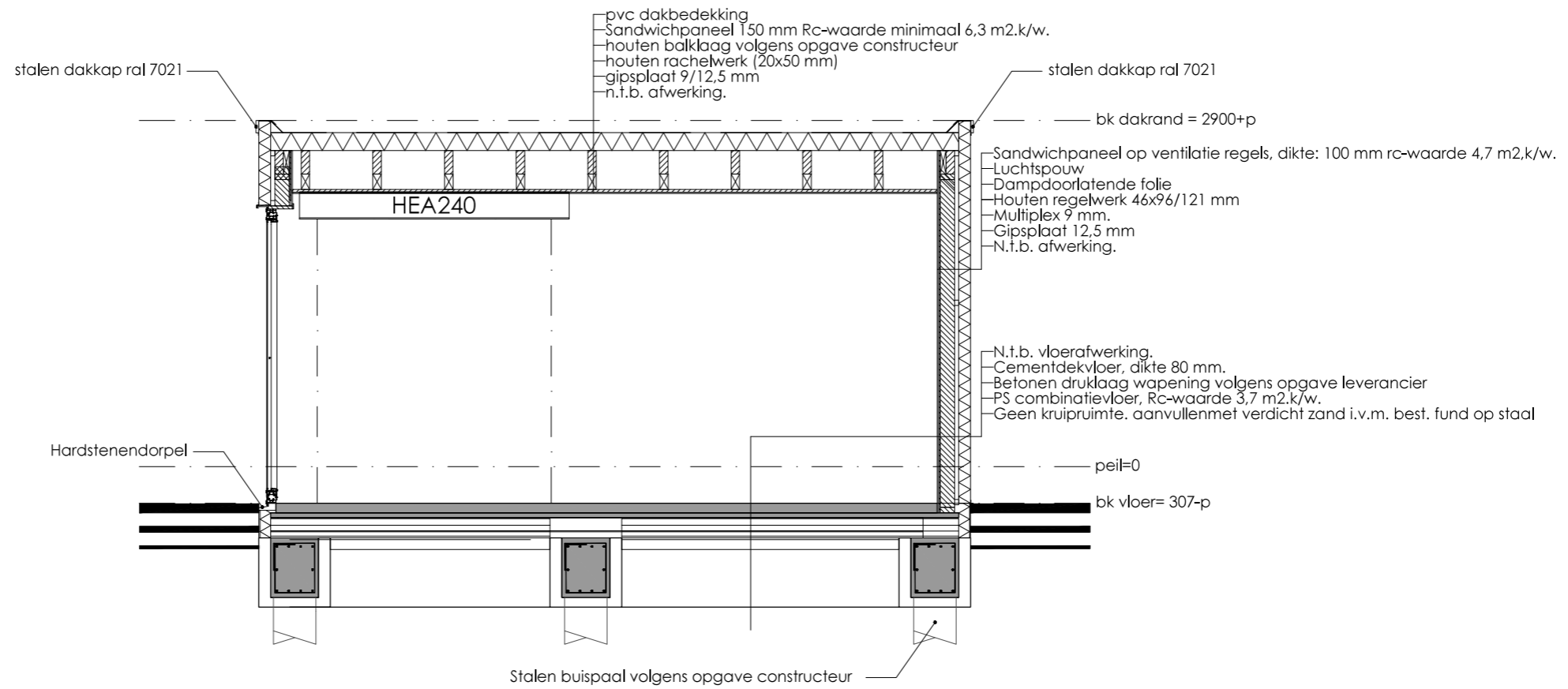
Doorsnede B-B (bij pui)
