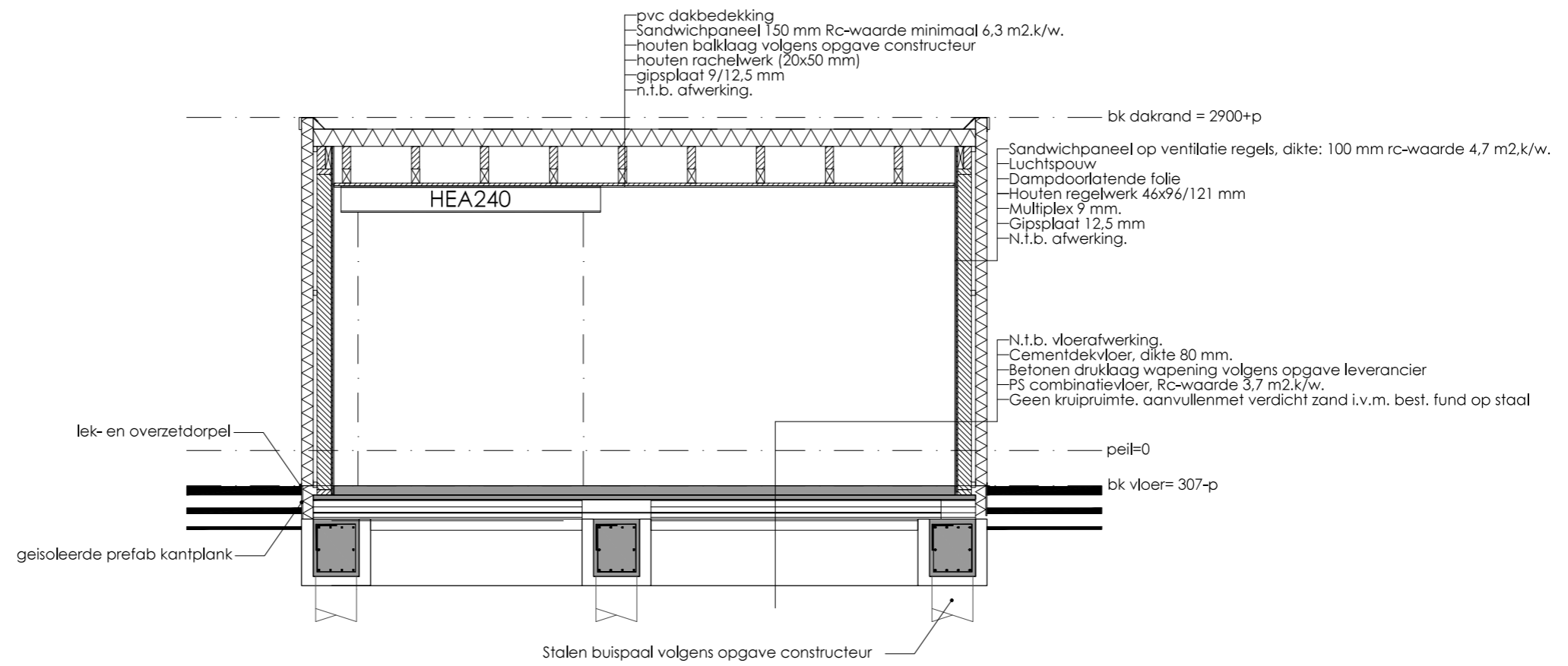
Doorsnede B-B (bij wand)
