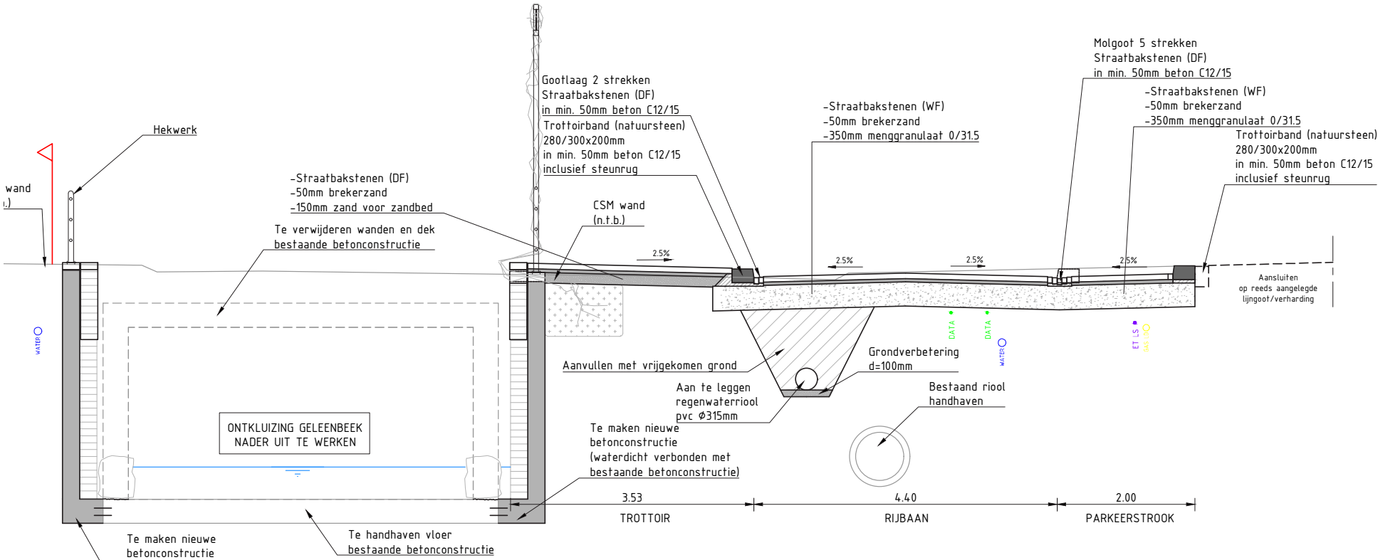
Doorsnede Parklaan tussen Engelenkampstraat- Wilhelminastraat en Wieër
