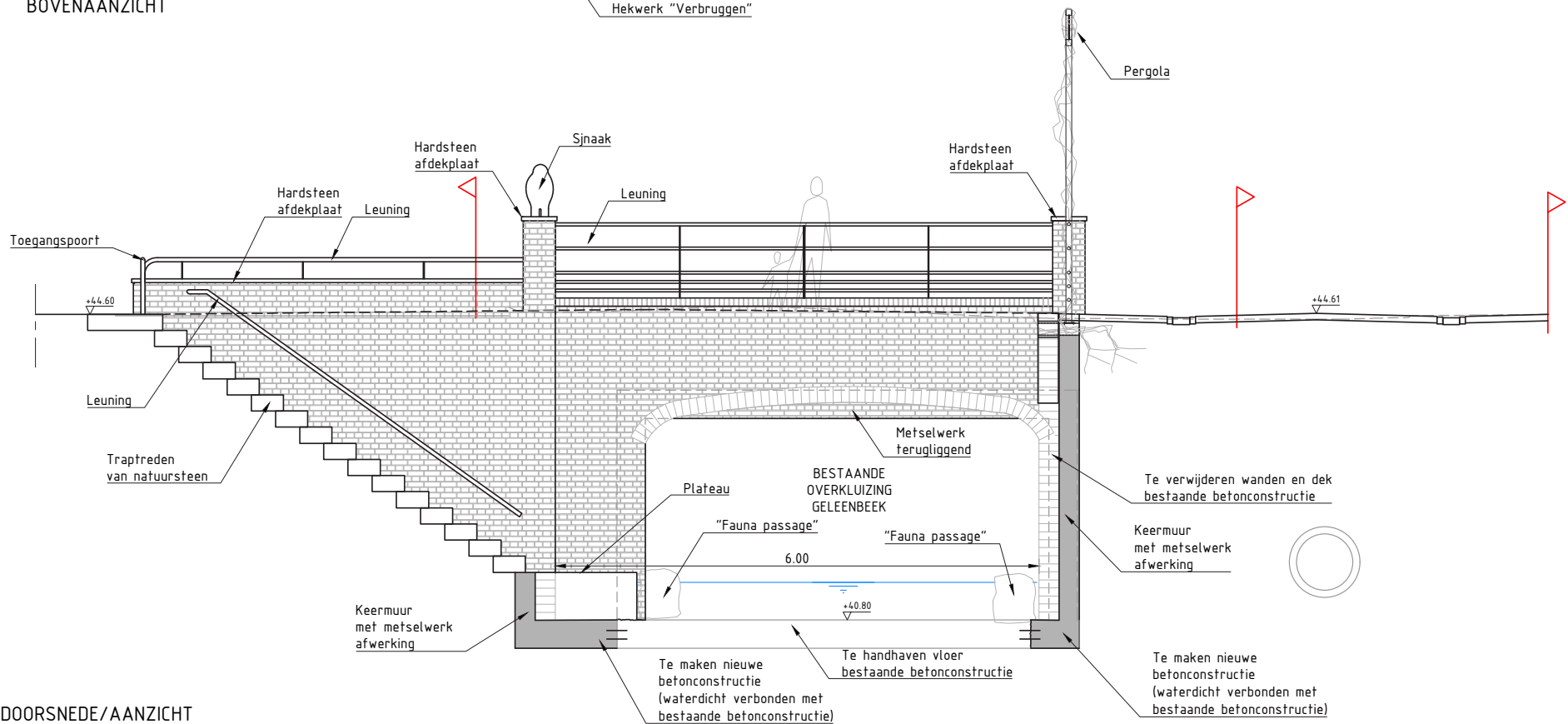
DOORSNEDE/AANZICHT
