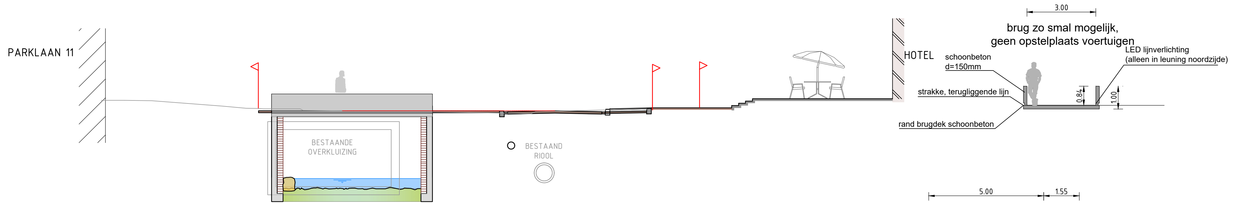
DWARSPROFIEL B9
