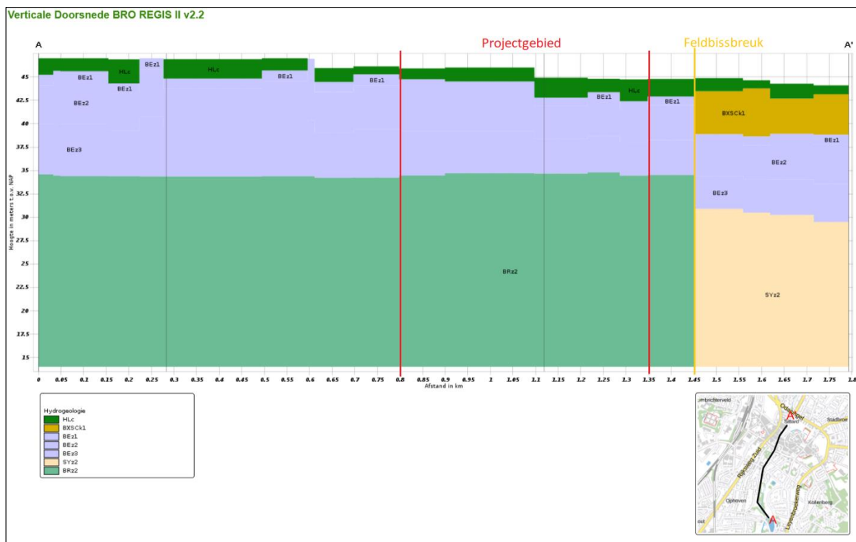
Figuur 3.1: Profiel REGIS
