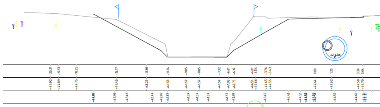
Figuur 7.1 Bestaande (lichtgrijs) en nieuwe (zwart) situatie
