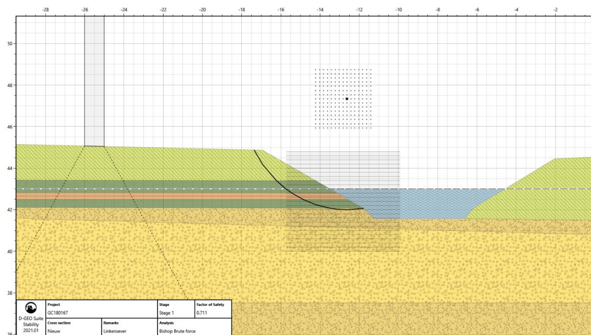
Figuur 7.1 Stabiliteitsberekening nieuwe situatie
