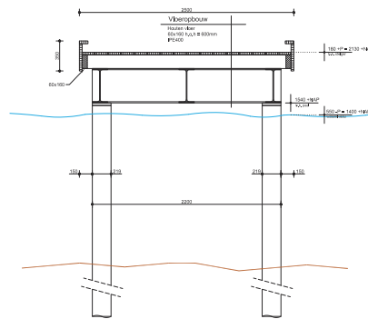
Doorsnede D-D
