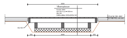
Doorsnede A-A
