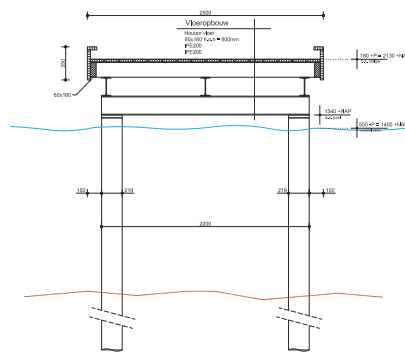
Doorsnede C-C
