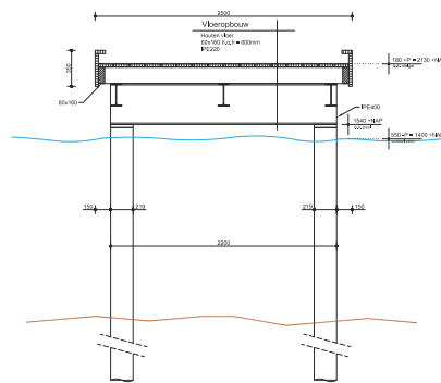
Doorsnede E-E
