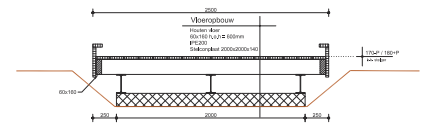
Doorsnede B-B
