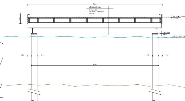
Doorsnede F-F
