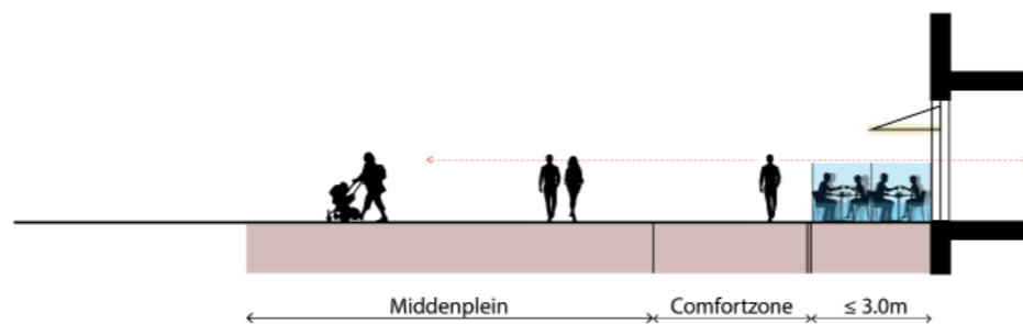
Afbeelding 6: Principeddoorsnede opstelling luifels gevelterras \leq 3 meter
