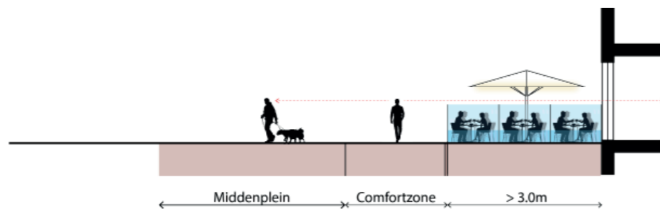
Afbeelding 7: Principeddoorsnede opstelling parasol gevelterras > 3 meter
