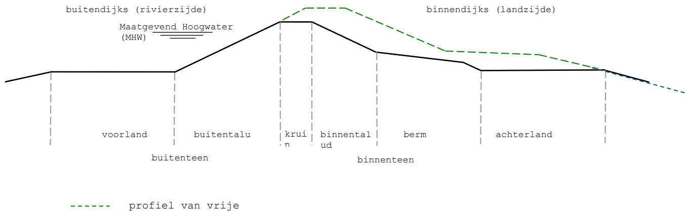
Figuur 1. waterkering met profiel van vrije ruimte
