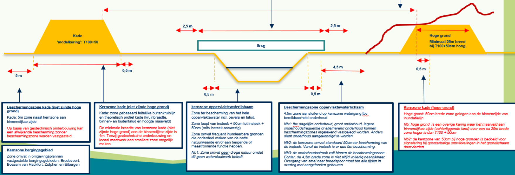
figuur 2.1 schematische weergave van de kernzone en beschermingszone van een watergang en kade
