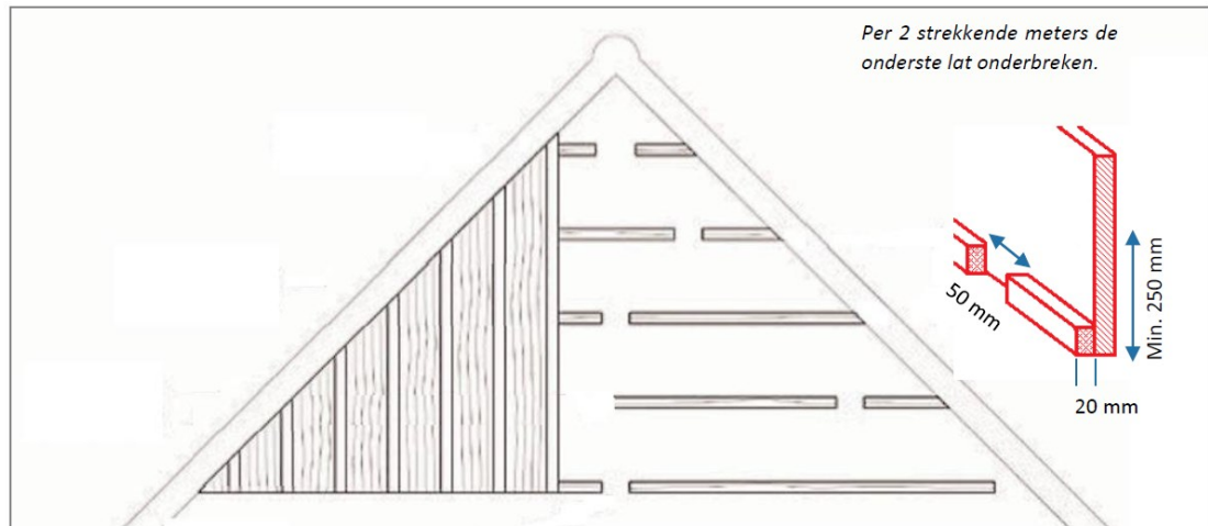
Afbeelding 2.3 | Detailtekening houten gevelbetimmering. Figuur 2: permanente voorzieningen (Viridis, 2022).
