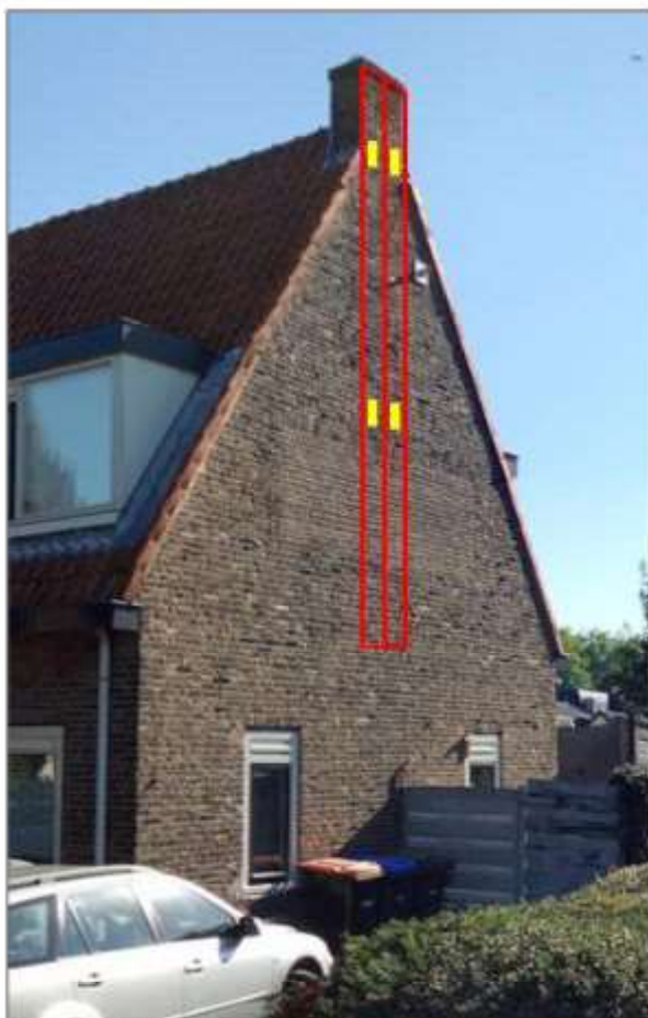
Figuur 3: Wijze van realisatie permanente voorzieningen voor laatvlieger. De schoorsteenkanalen (rood) worden, indien dit nog niet het geval is, aan zowel de bovenzijde als onderzijde afgesloten, ter hoogte van de bovenste kantpannen én halverwege de schoorsteen worden in totaal 4 open stootvoegen gemaakt om laatvlieger toegang te geven tot de schoorsteenkanalen.
