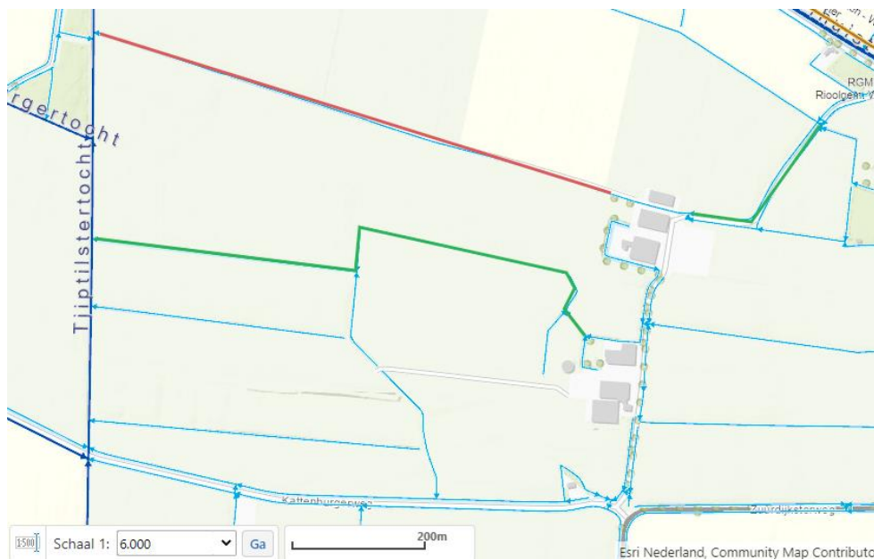
Figuur 1: Locatie kadastraal bekend LEE02L738. De groene lijnen geven de te verbreden secundaire watergangen weer, de rode lijn is de te dempen secundaire watergang
