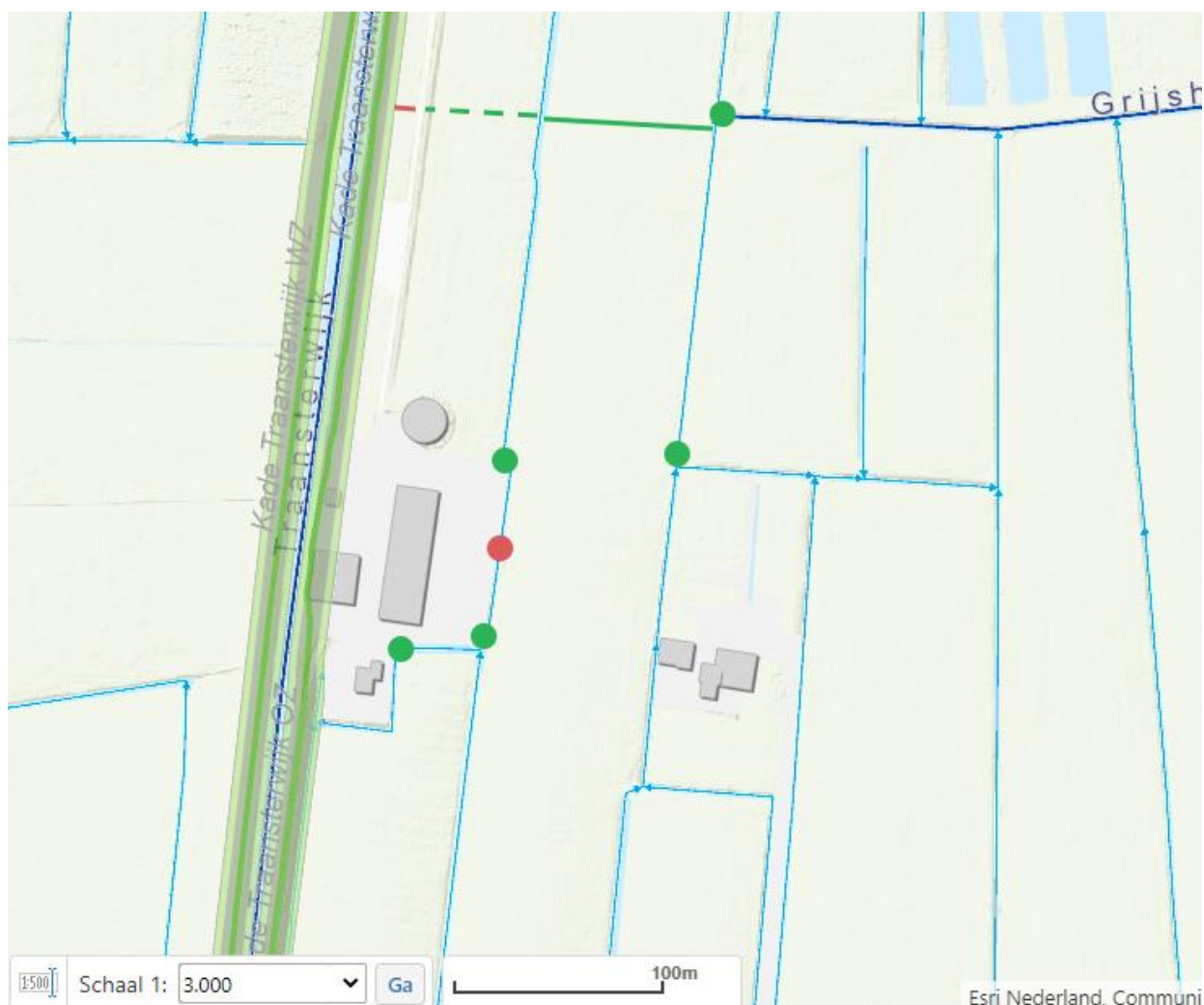
Figuur 1: Schematische tekening van de werkzaamheden. De groene stippen geven de locatie weer van de aan te brengen duikers in bestaande dammen. De rode stip geeft de locatie weer van de te verwijderen dam. De groene lijnen zijn te graven watergangen en de rode lijn geeft de locatie weer van het te plaatsen schapengaas met palen en hekwerk.
