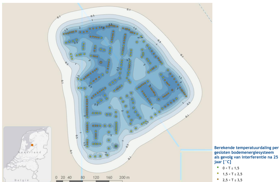
Figuur 3.1 | Thermische beïnvloeding tussen 0 en 225 m-mv na 25 jaar (zie ook Bijlage 1 voor groot formaat)
