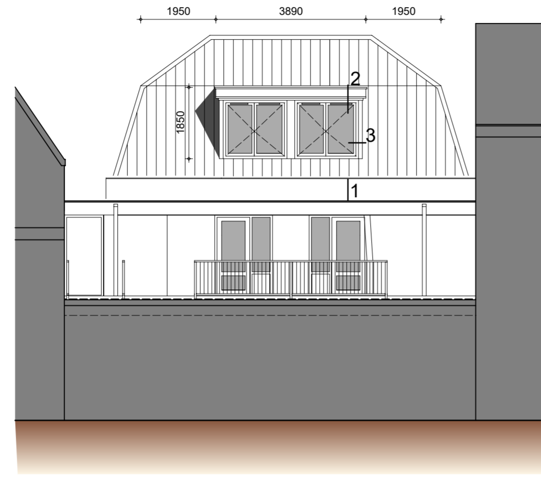
Achtergevel Van der Werfstraat
