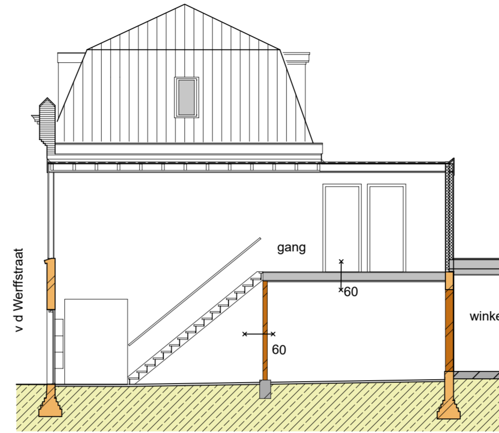
Rechter zijgevel Van der Werfstraat
