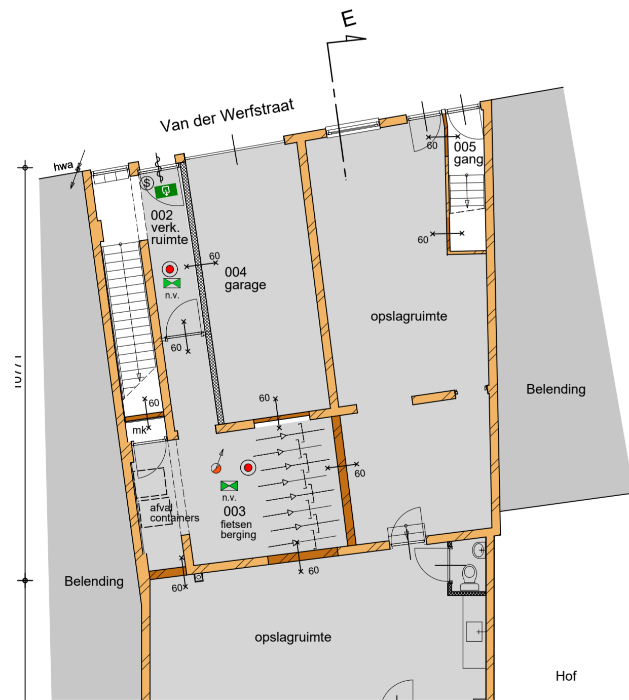
Begane grond (ongewijzigd)
