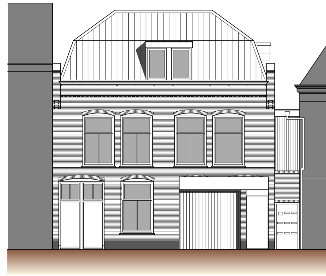
Voorgevel Van der Werfstraat
