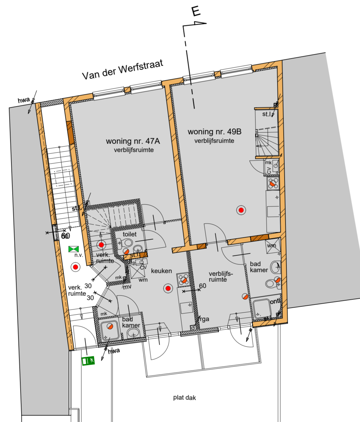
1e verdieping (ongewijzigd)
