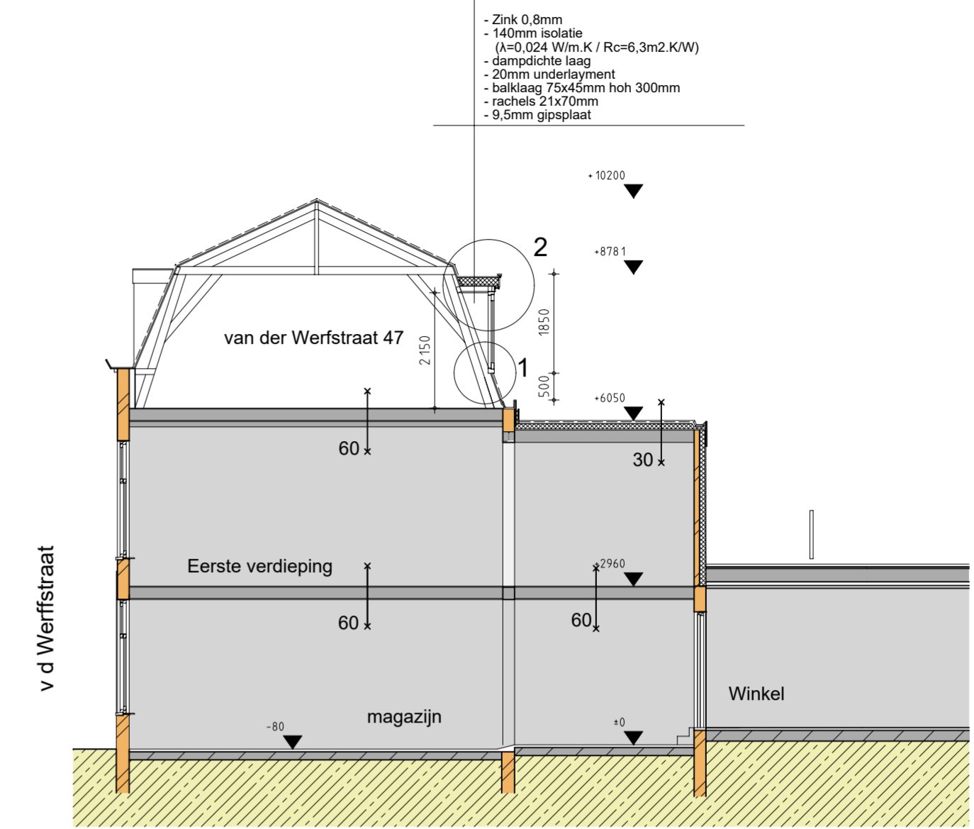
Langsdoorsnede E - E
