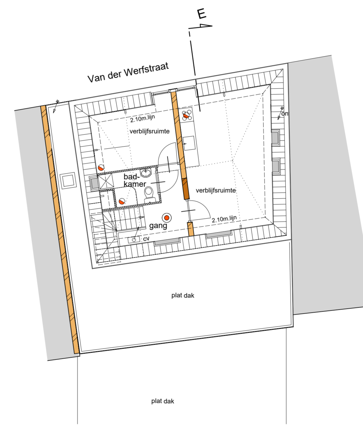
2e verdieping
