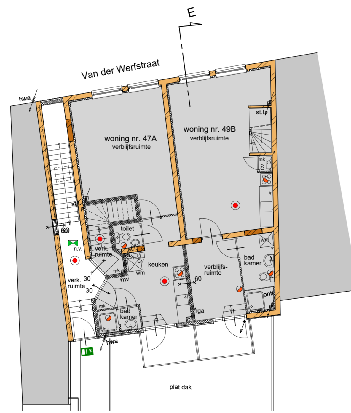
1e verdieping
