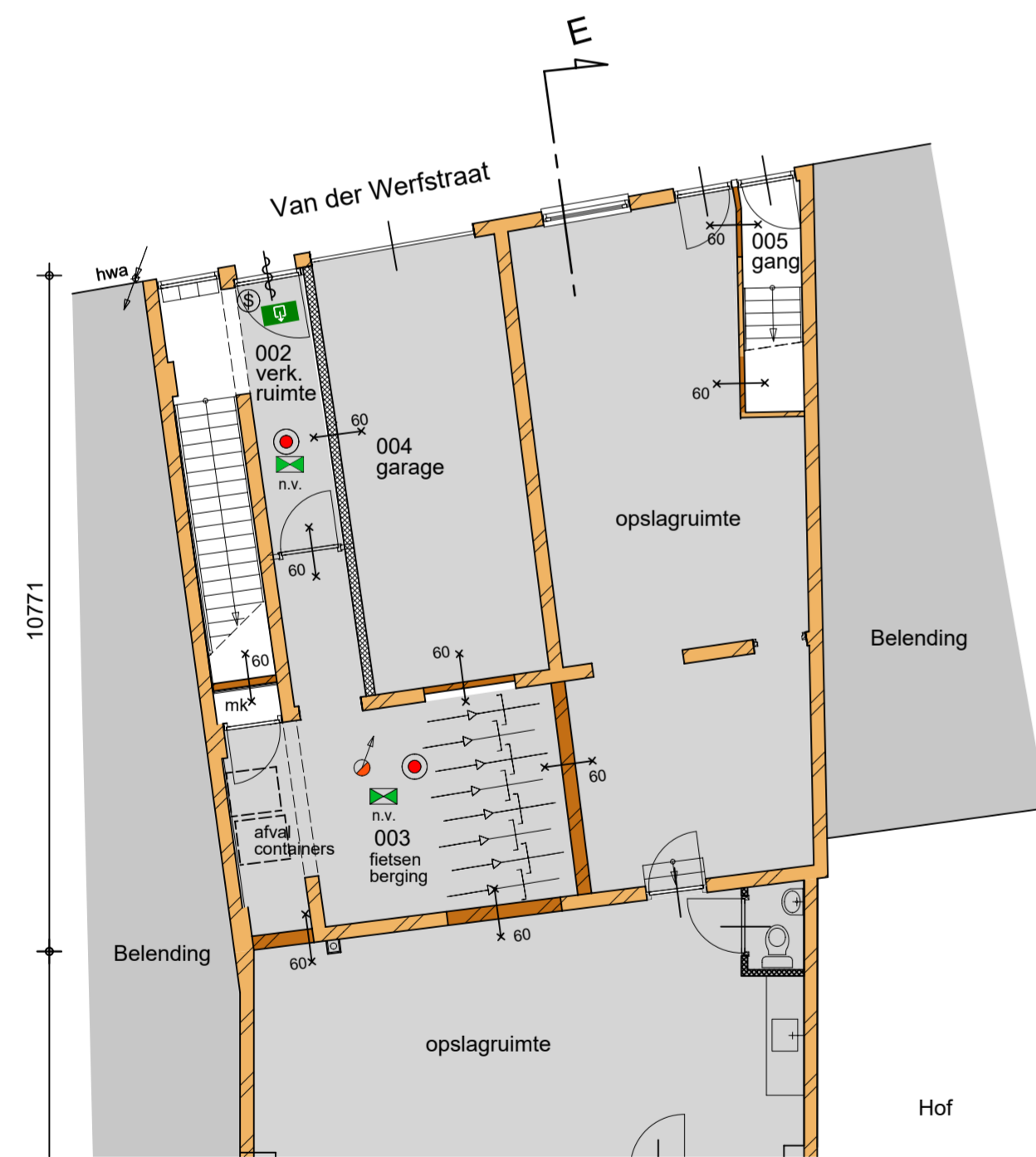
Begane grond
