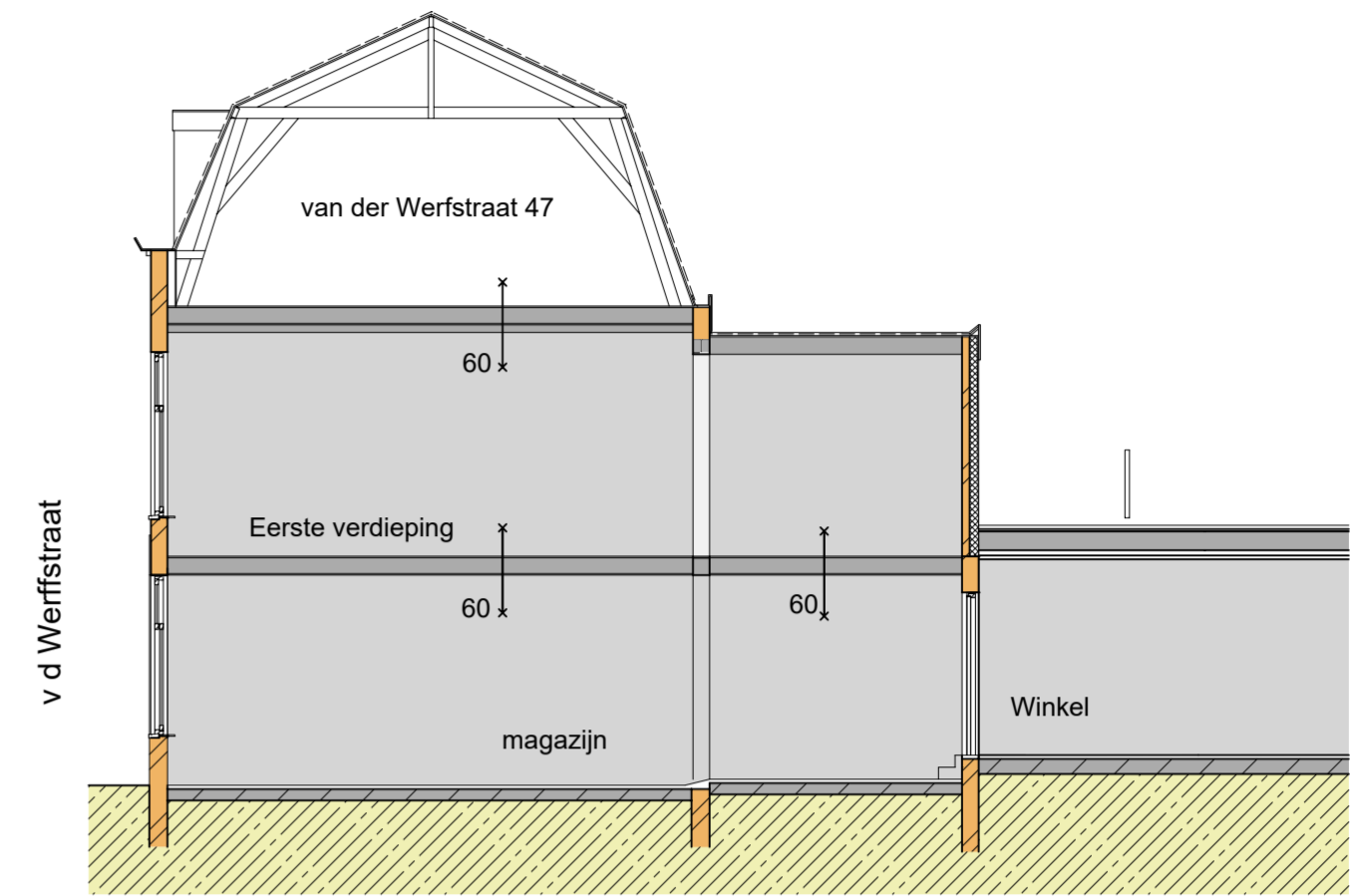
Langsdoorsnede E - E
