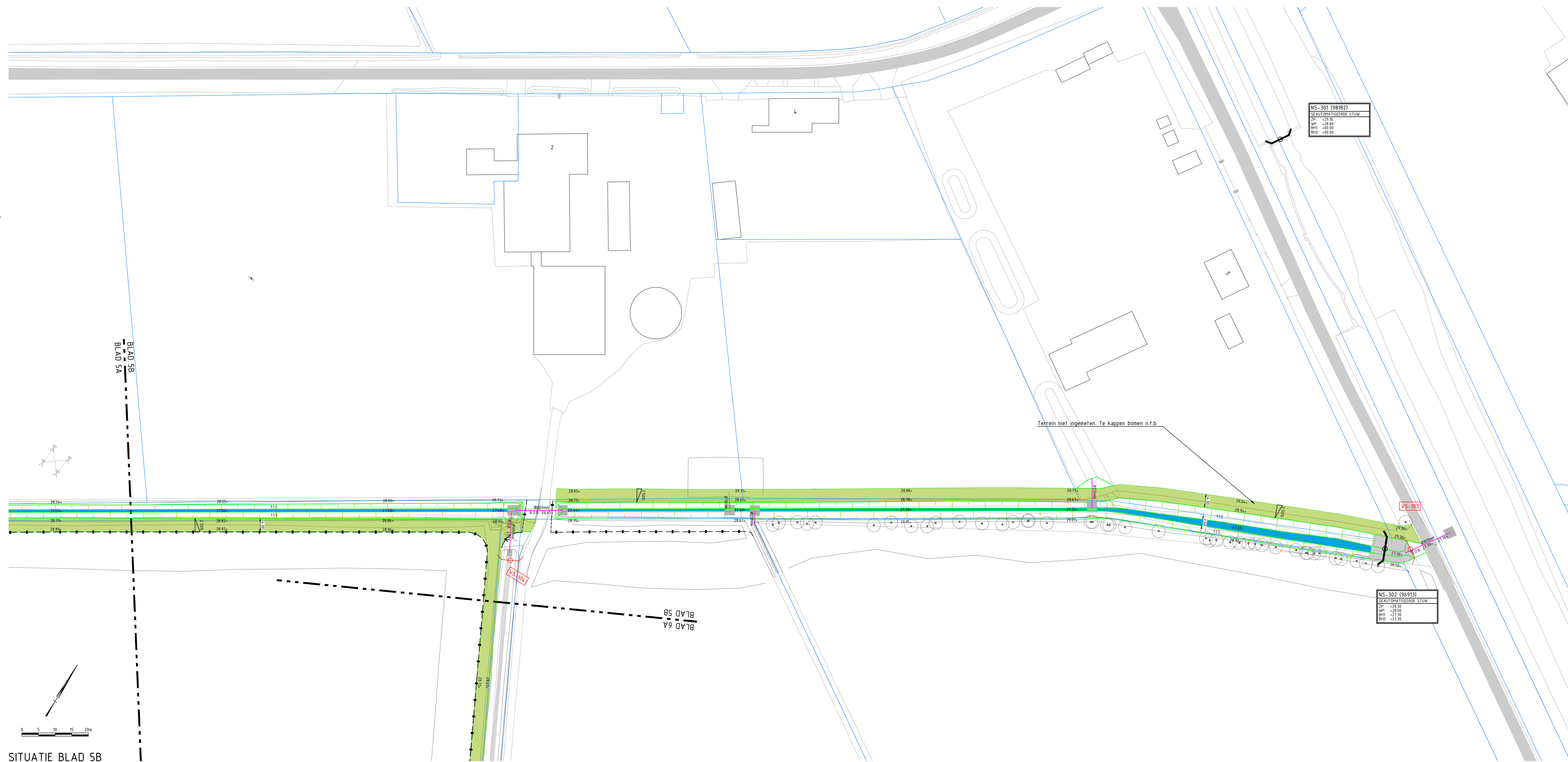
SITUATIE BLAD 5B SCHAAL 1:500
