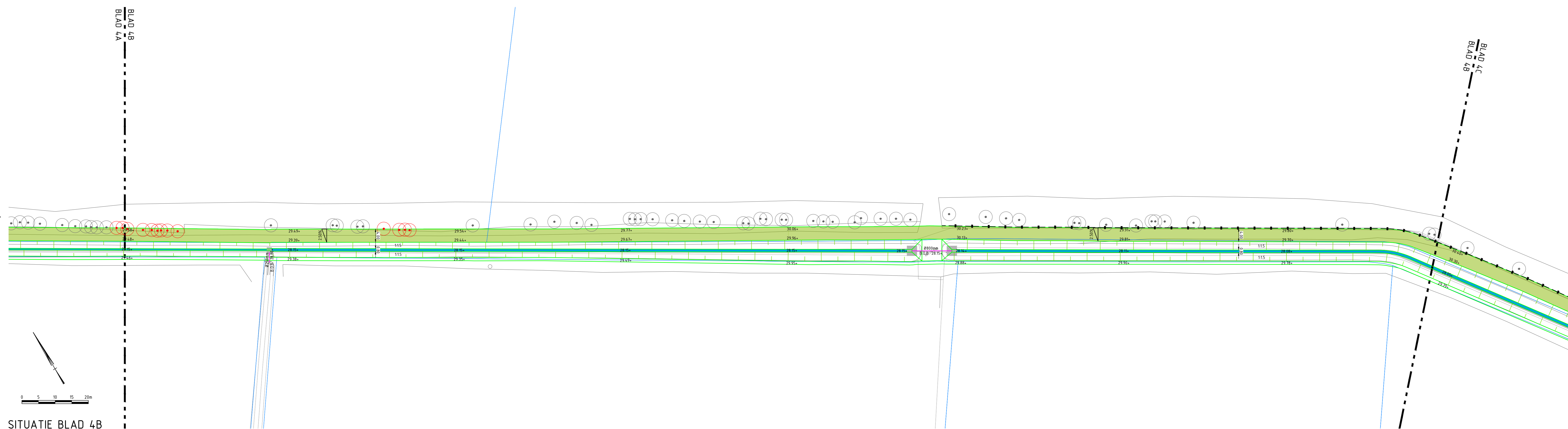
SITUATIE BLAD 4B SCHAAL 1500
