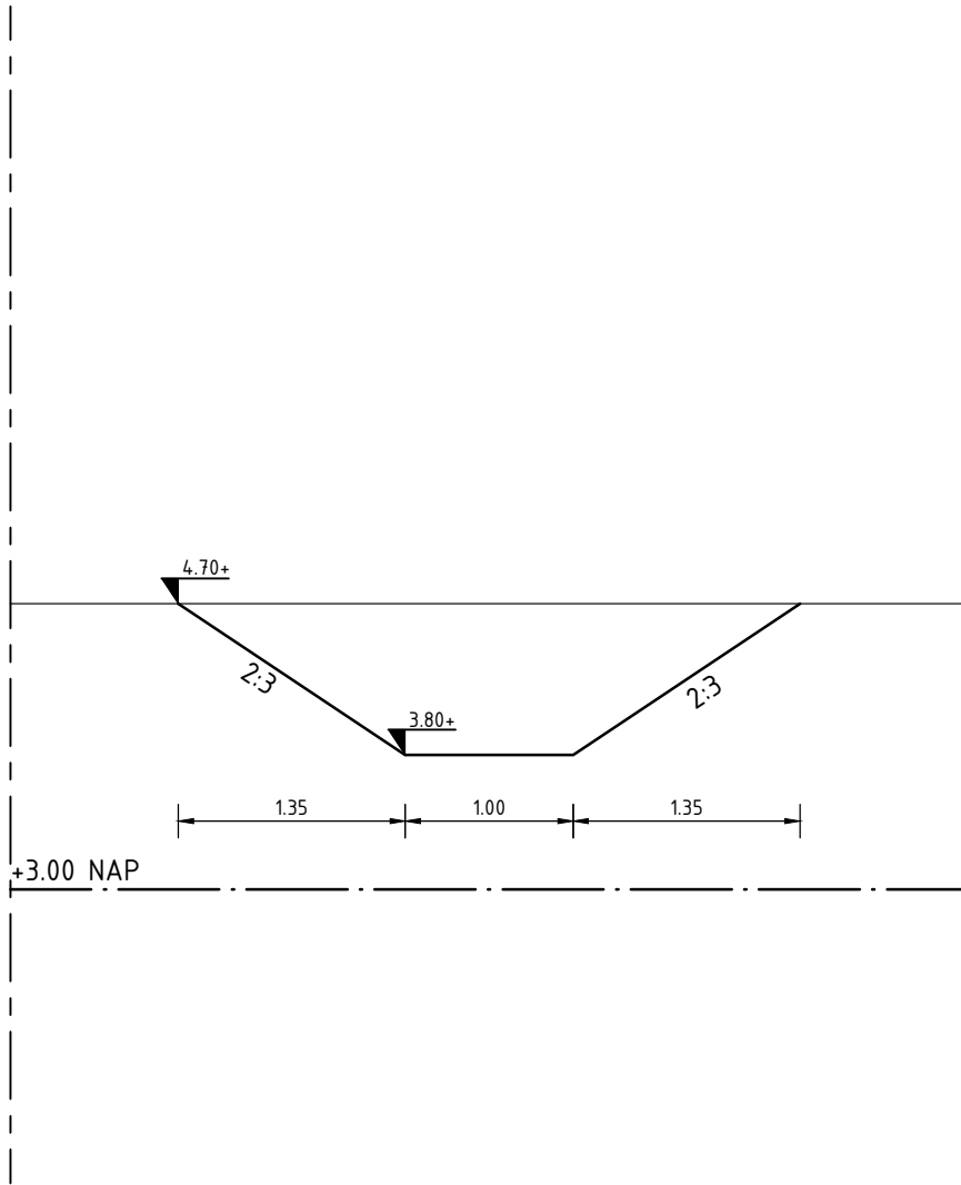
Doorsnede G-G Schaal 1:50
