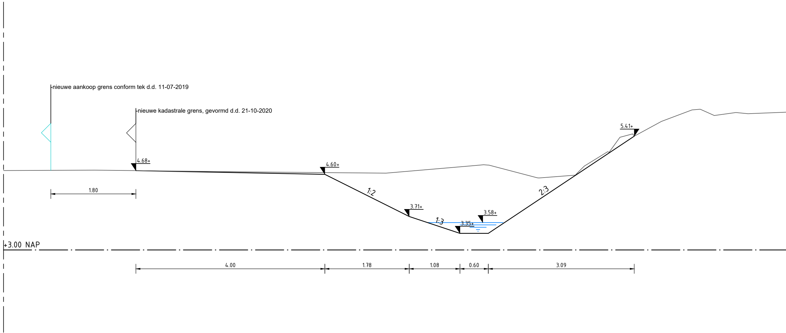
Doorsnede C-C Schaal 1:50
