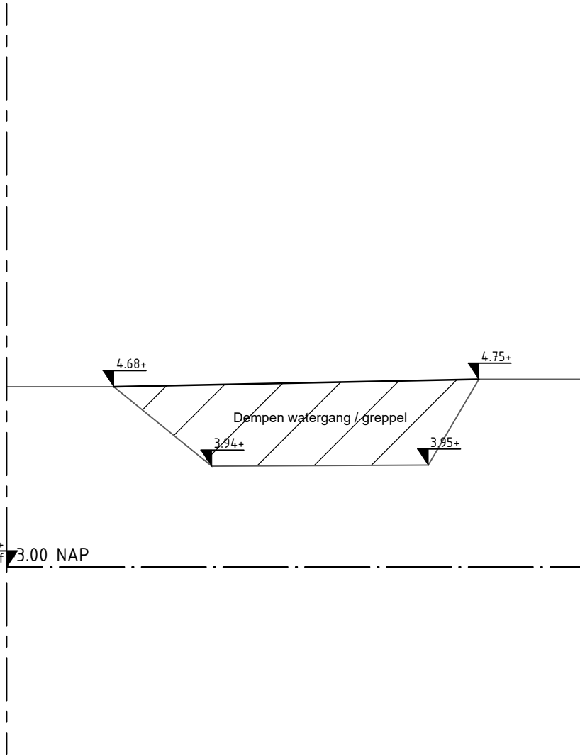
Doorsnede H-H Schaal 1:50
