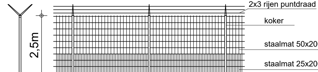
principe hekwerk
