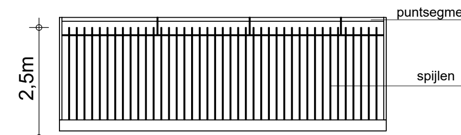
principe poort
