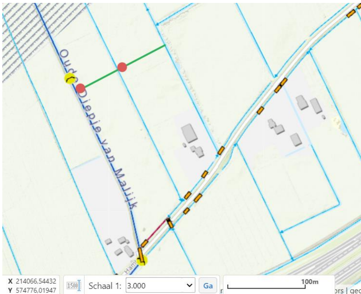
Figuur 1: Globale locatie van de werkzaamheden. De groene lijn geeft de nieuw te graven watergang weer, de rode stippen zijn de aan te brengen dammen met duiker.
