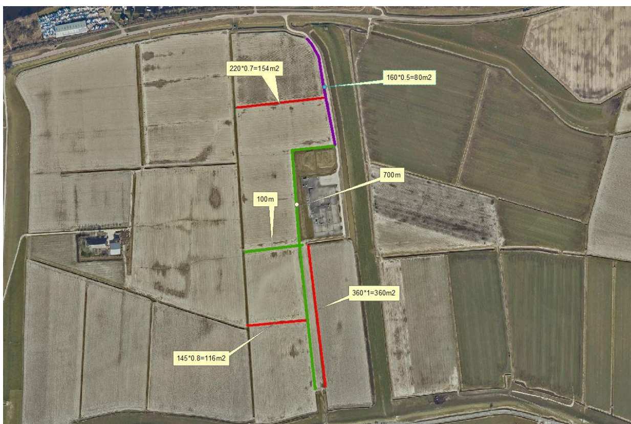
Figuur 1: De rode lijnen zijn de te dempen watergang, de groene lijnen zijn de te verbreden watergangen en de paarse lijn geeft een nieuw te graven watergang weer.
