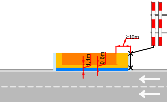
Werkvakindeling GOW
