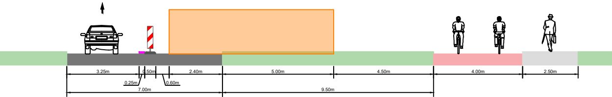
Dwarsdoorsnede A-A
