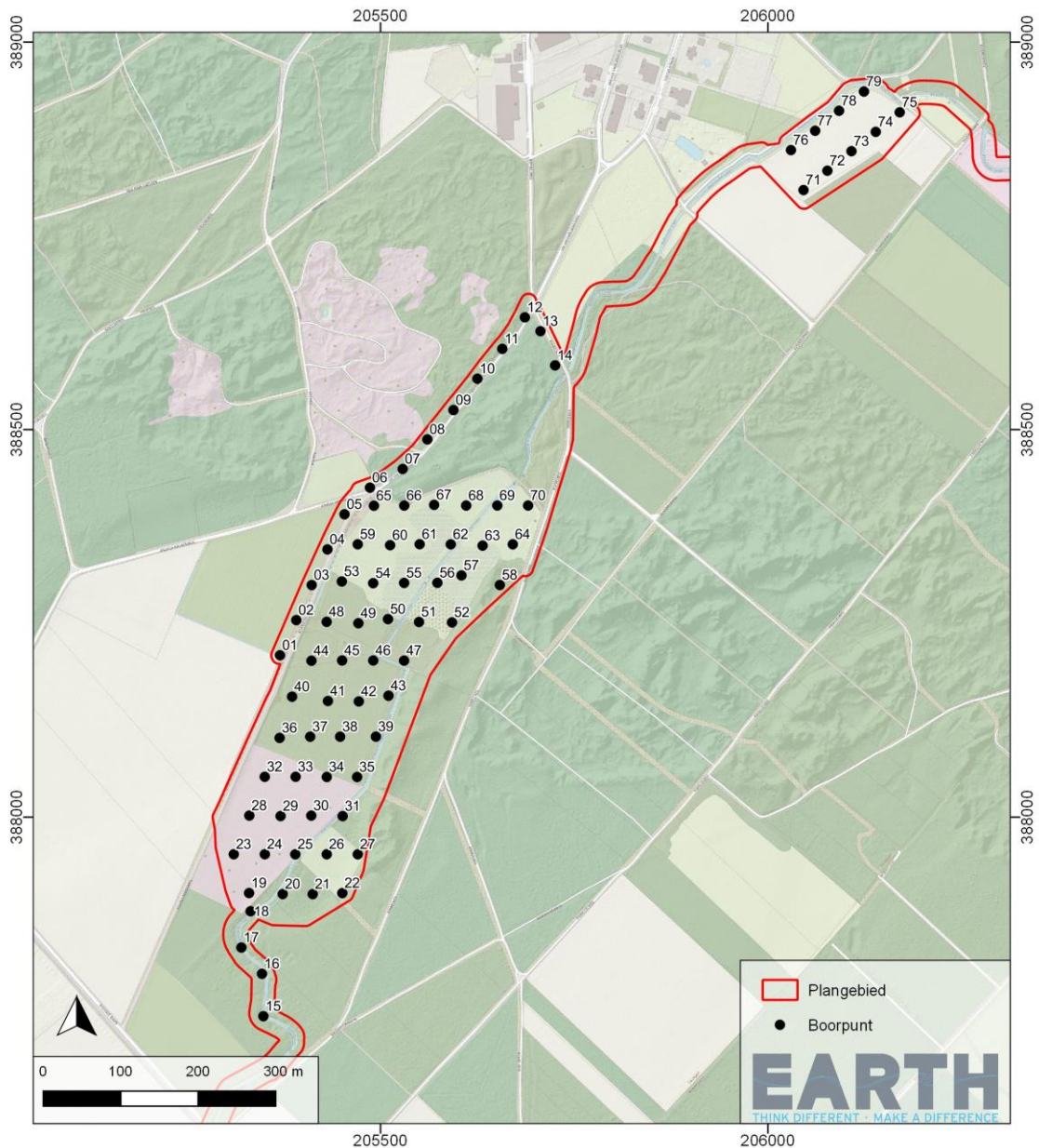
Afbeelding 4: Boorpuntenkaart van het verkennend booronderzoek.
