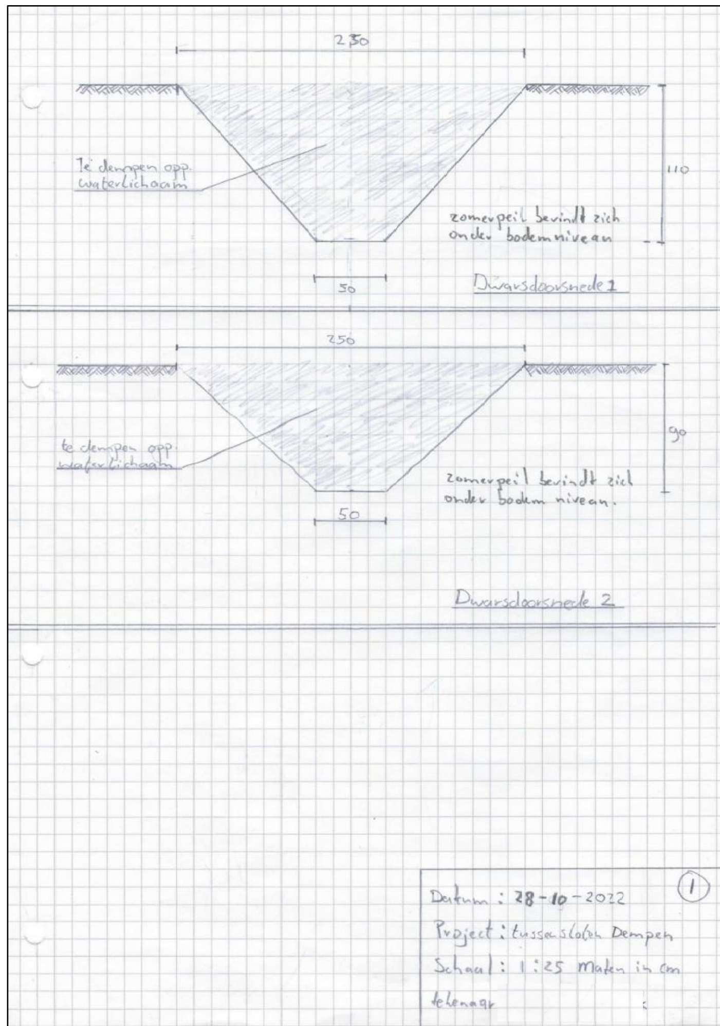
572293-C2 dwarsprofielen (dempen B-wateren en vergraven A-wateren)
