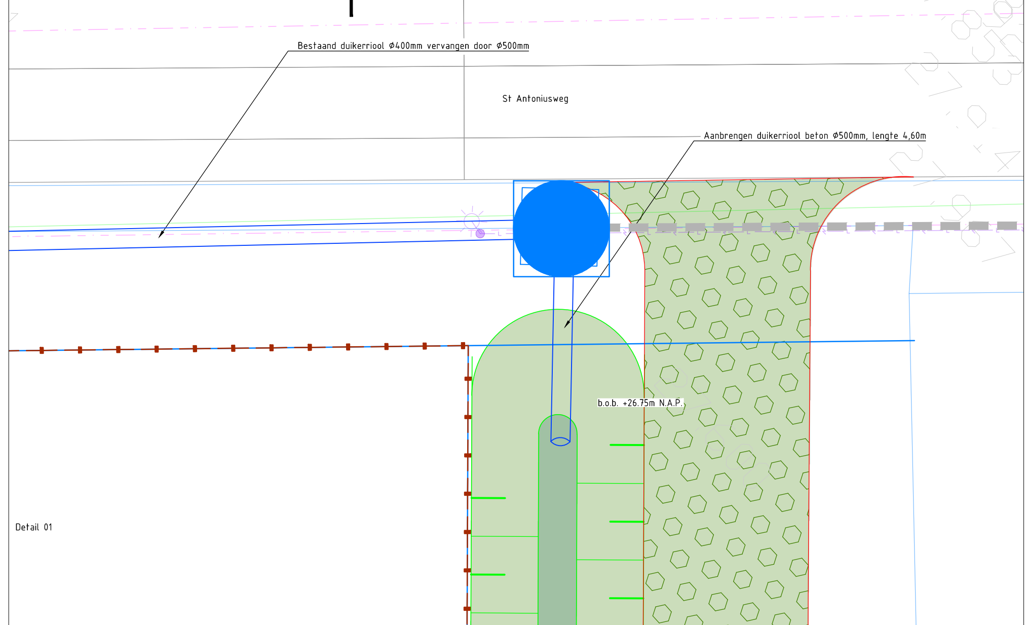
Detail: 01 Schaal 1:100
