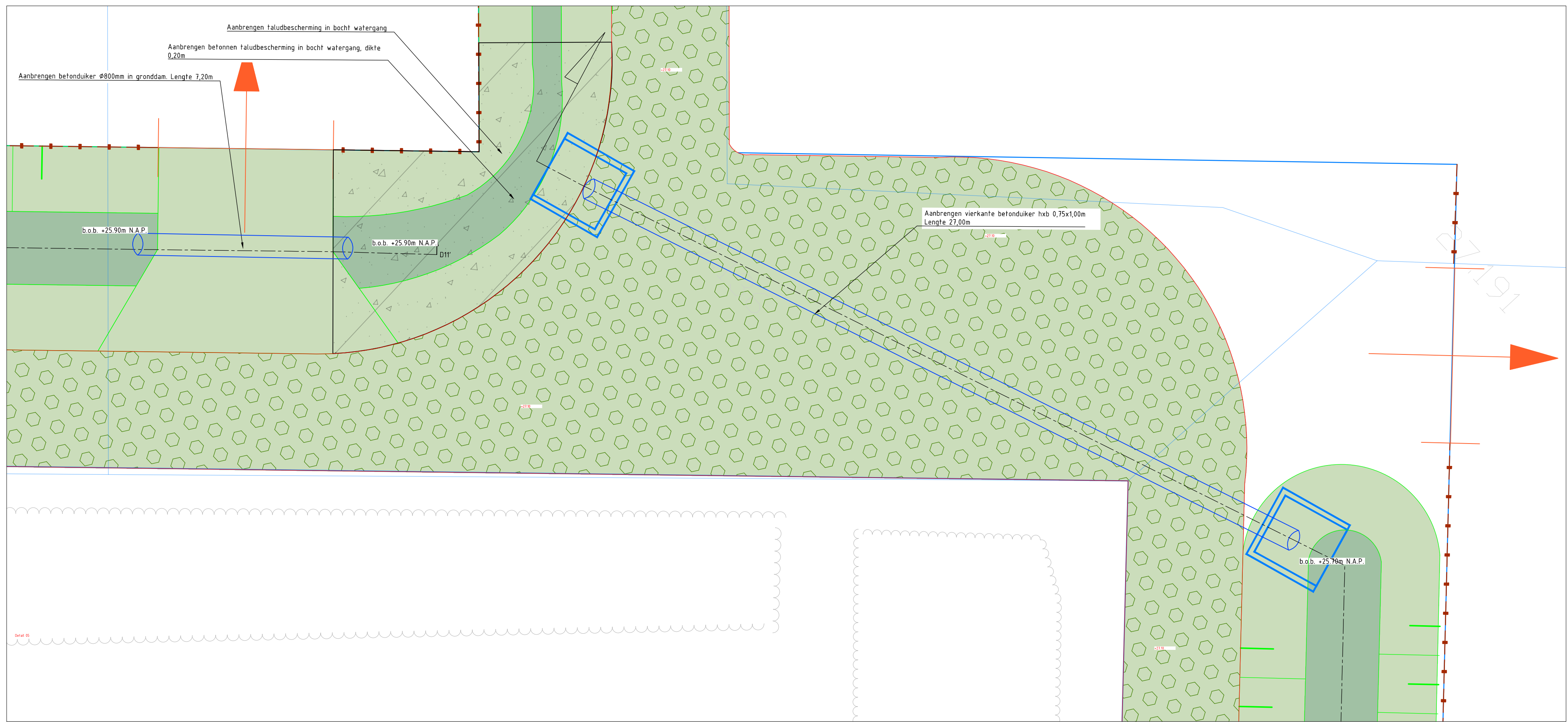
Detail: 05 Schaal 1:100
