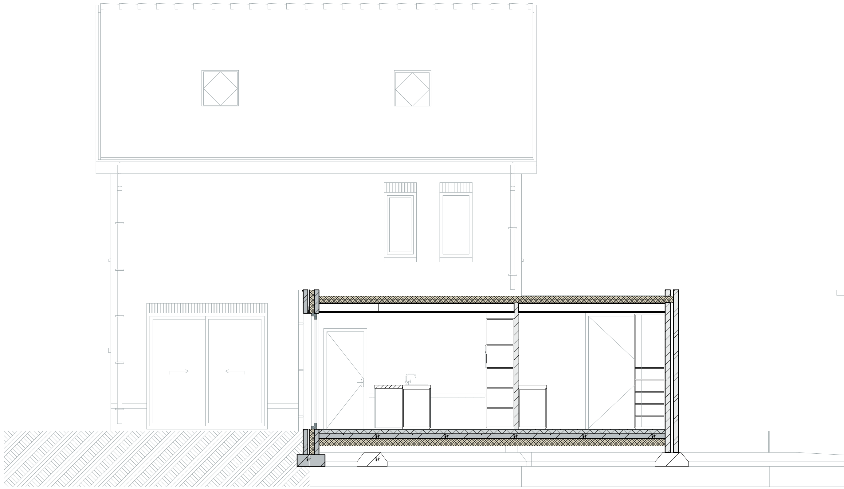
DOORSNEDE C-C
