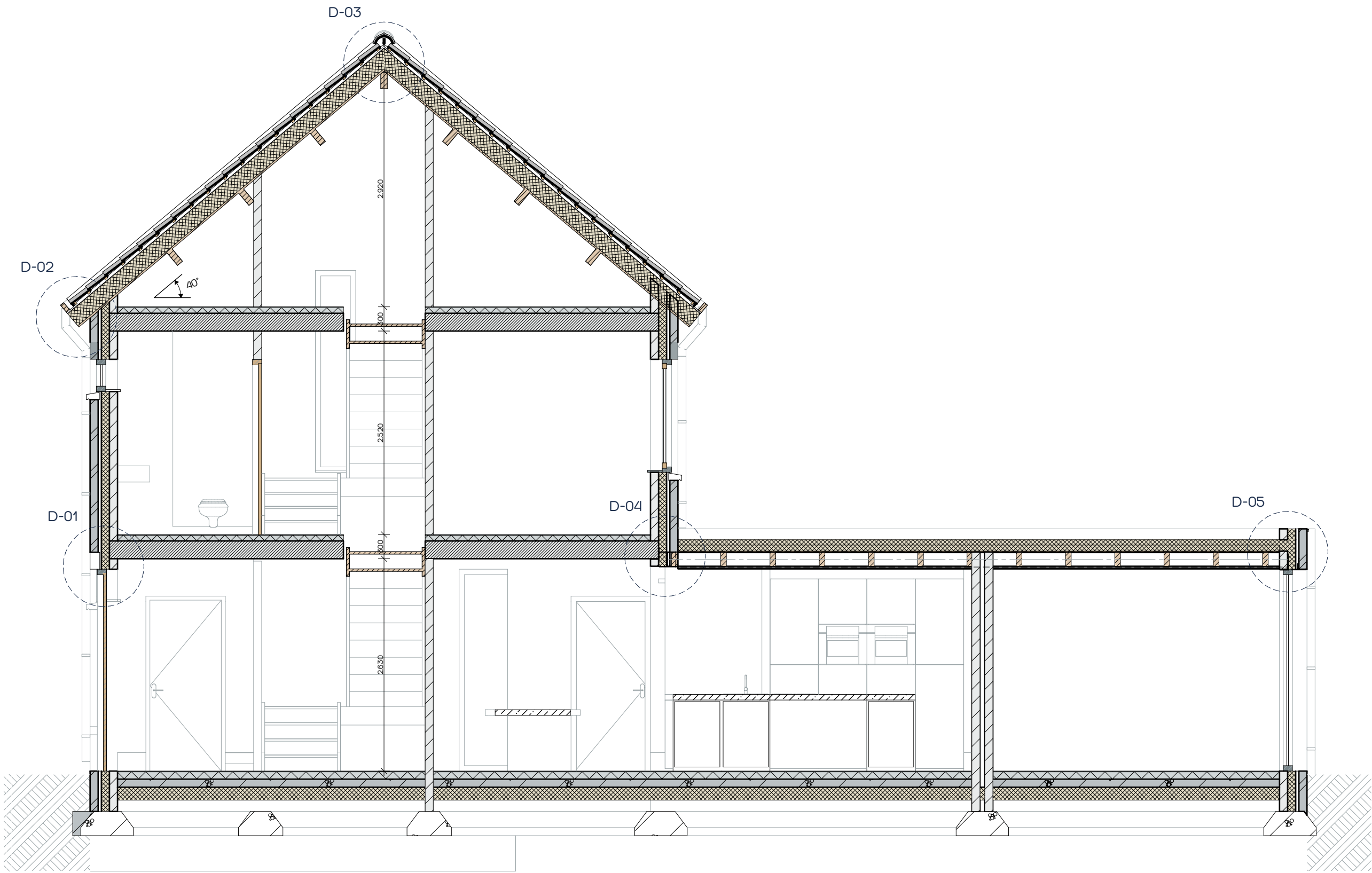
DOORSNEDE A-A
