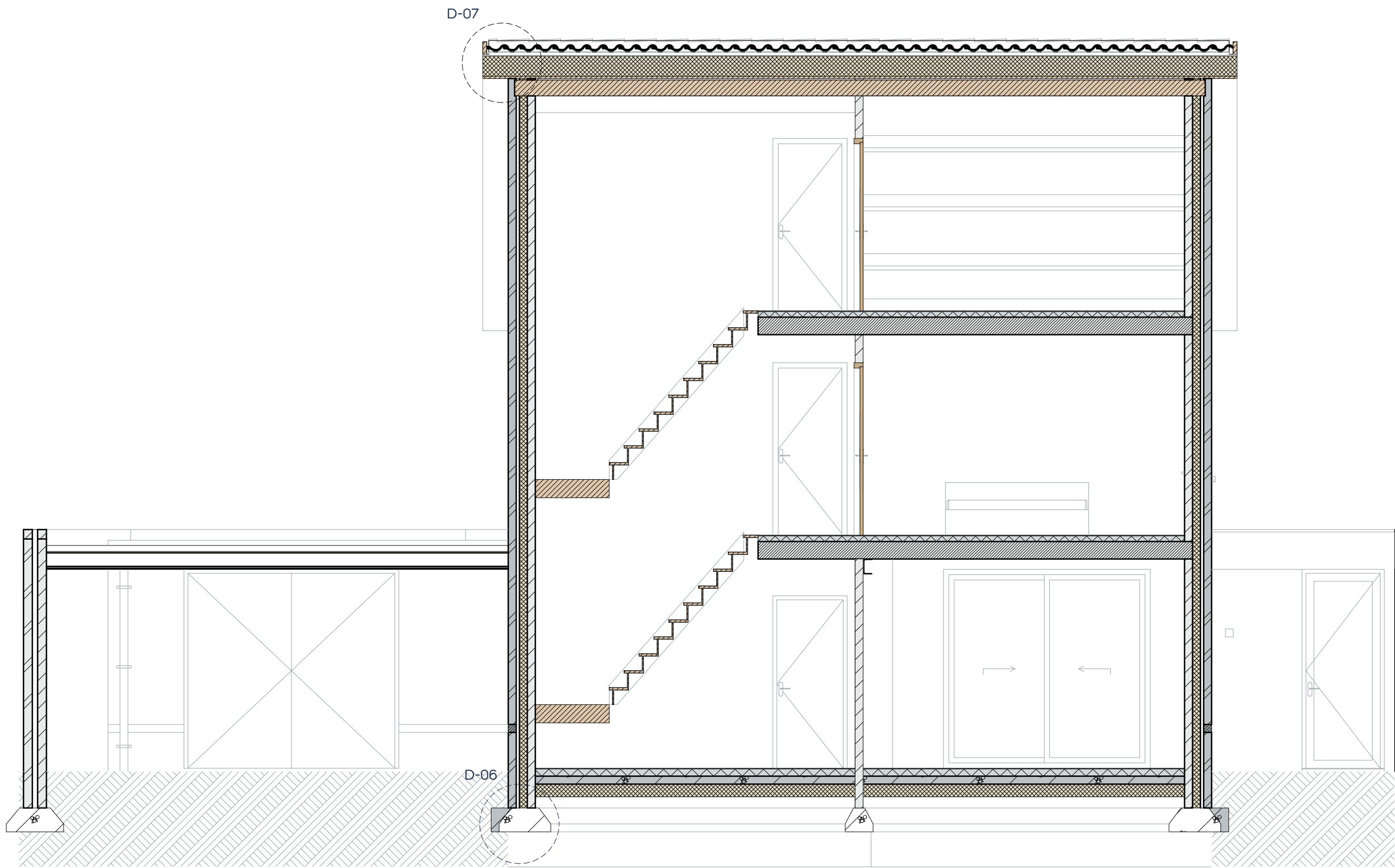
DOORSNEDE B-B
