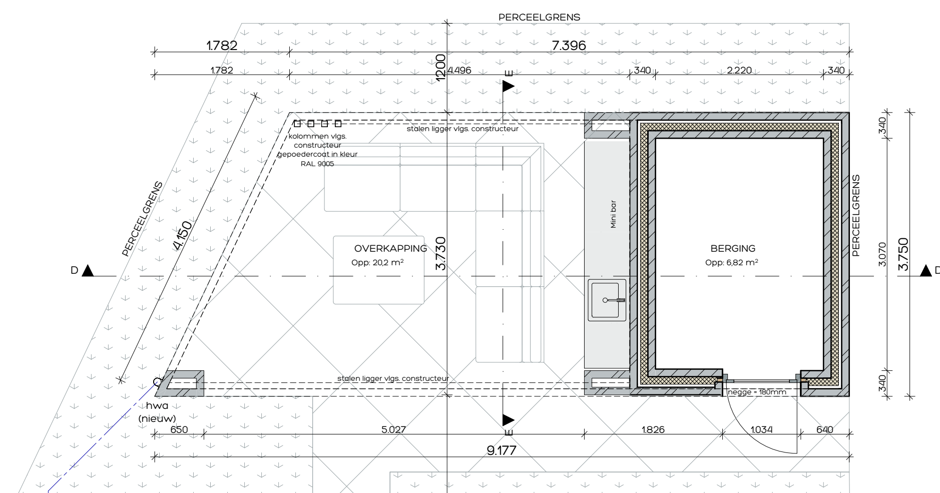
BEGANE GROND
