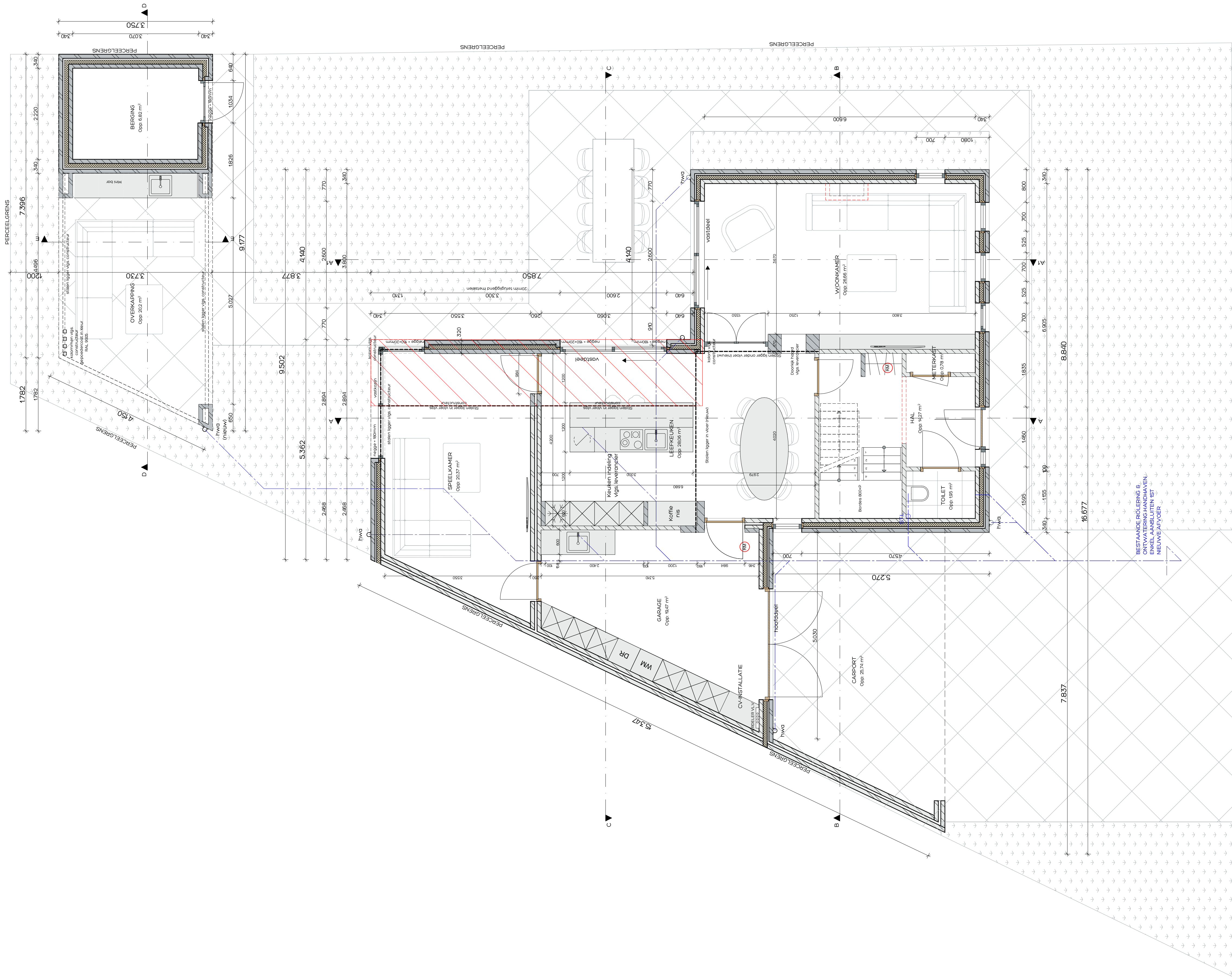
BEGANE GROND
