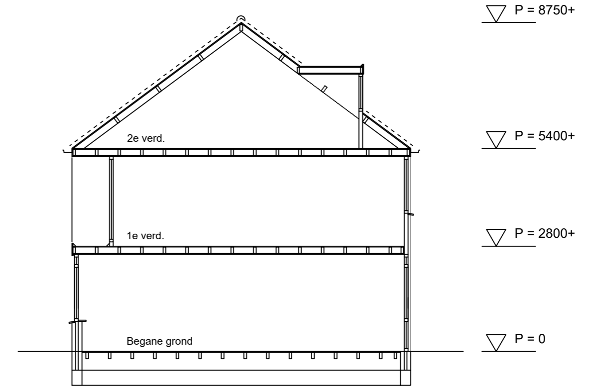
Doorsnede Bestaande situatie
