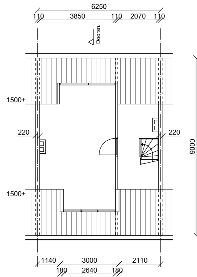
Plattegrond 2e verd. Nieuwe situatie
