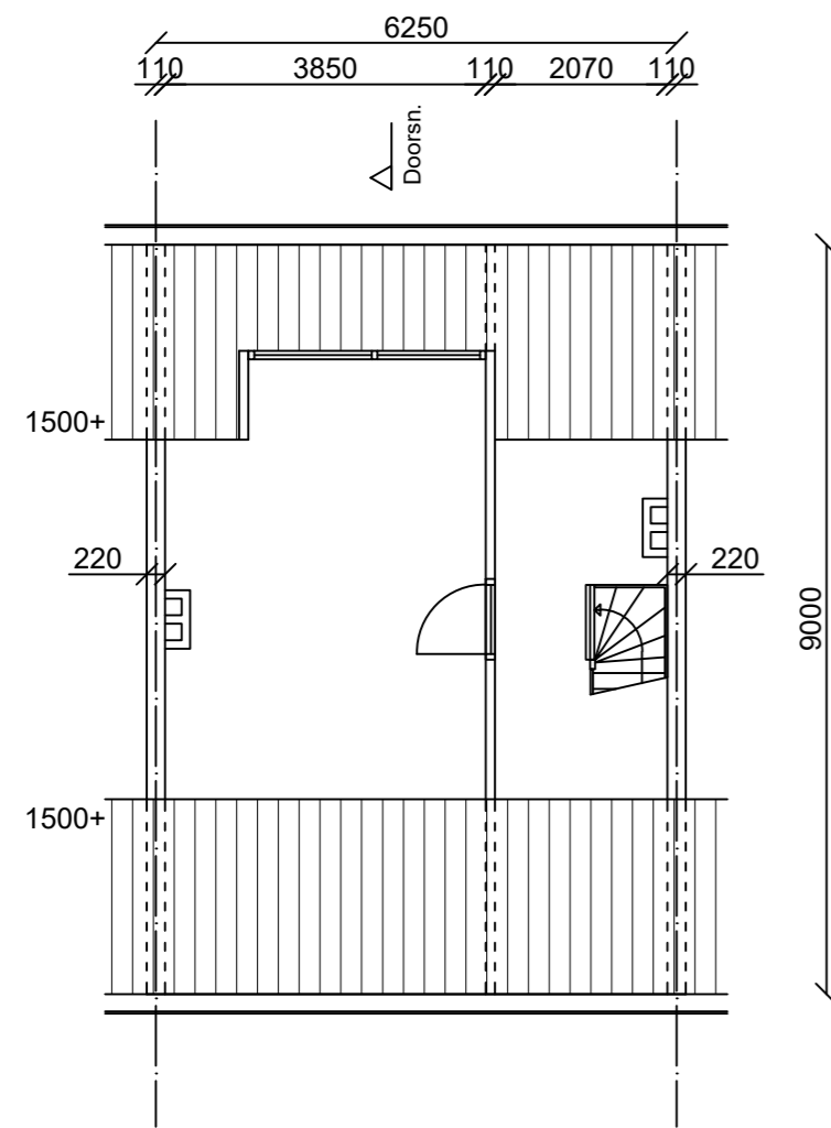
Plattegrond 2e verd. Bestaande situatie
