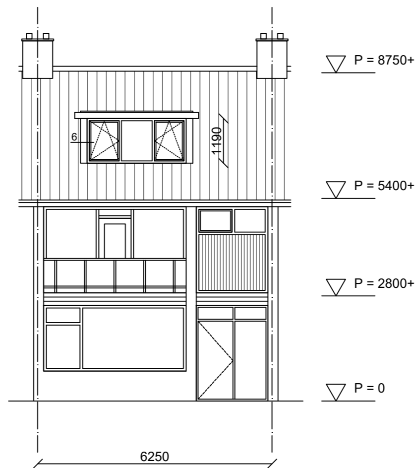
Vooraanzicht Nieuwe situatie
