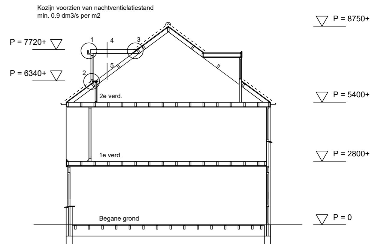
Doorsnede Nieuwe situatie
