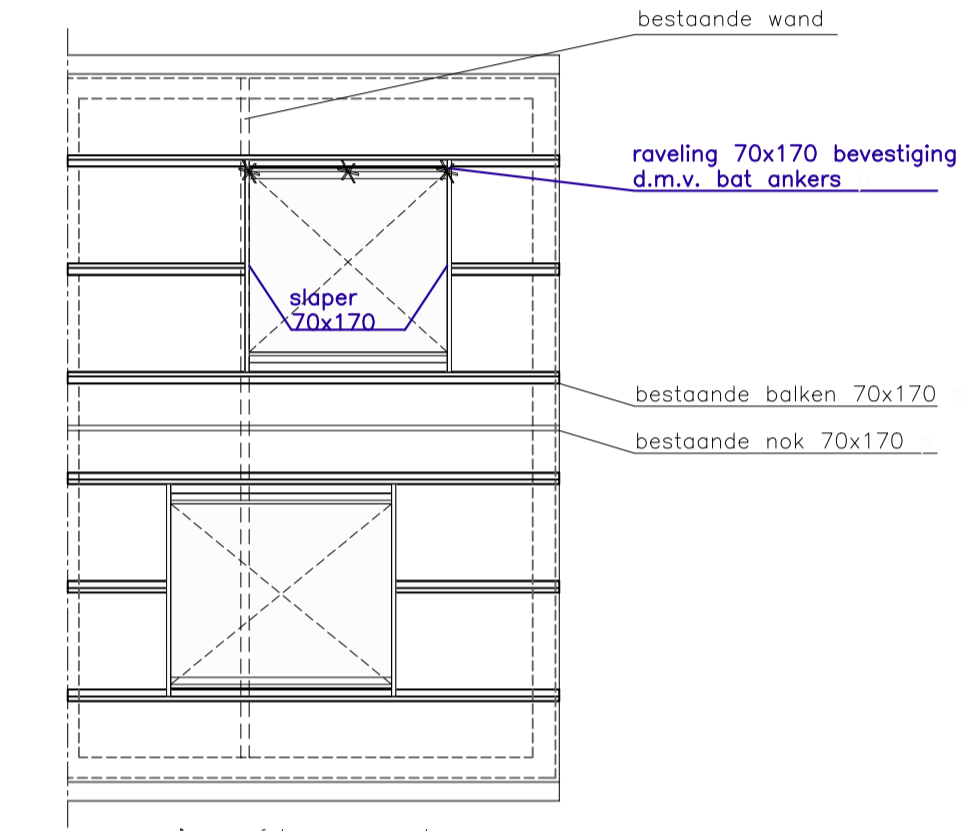
KAPPLAN NIEUW
