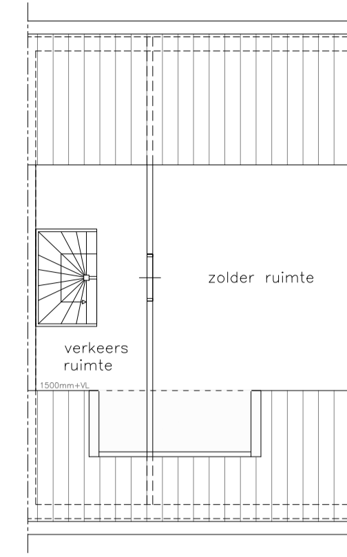
INDELING BESTAAND
