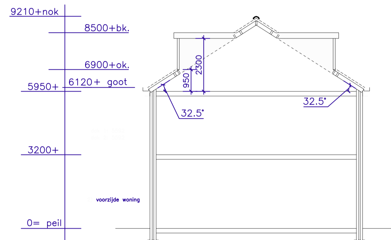
DOORSNEDE NIEUW
