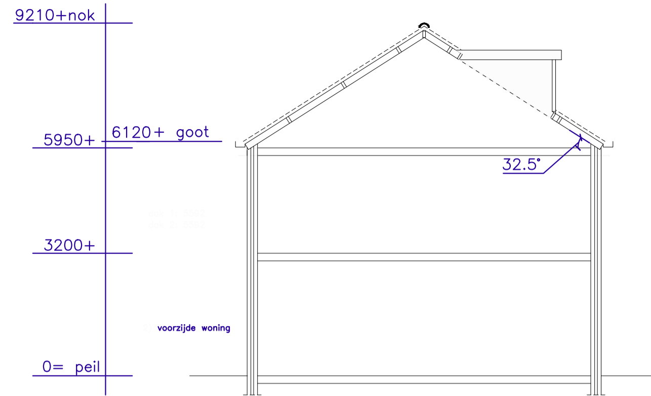
DOORSNEDE BESTAAND
