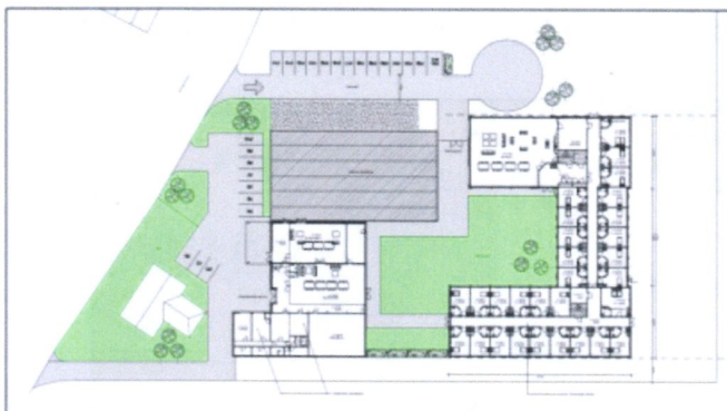
Figuur 2. Ontwerptekening toekomstige situatie
