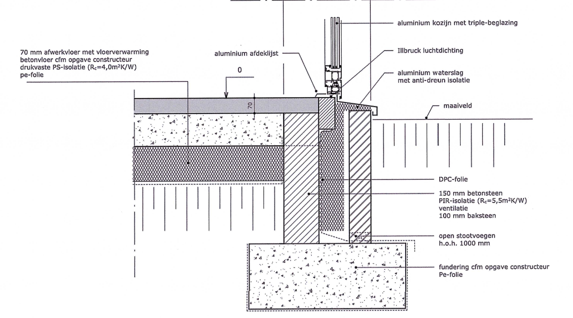
A - detail 1 1 : 10
