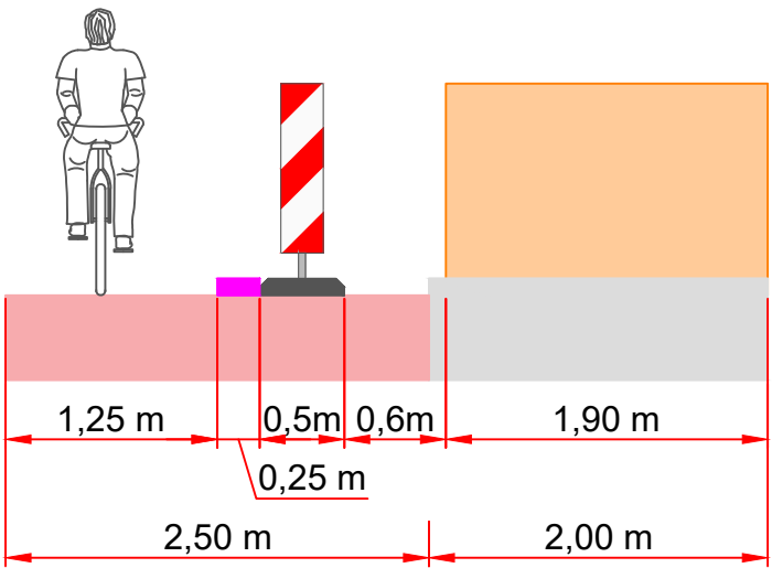
Dwarsdoorsnede A-A
