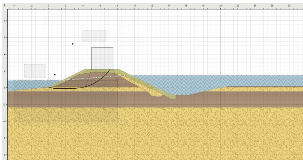
Figuur B2.1.2: Dijkvak 9A, STBI VO, variant met versterking in grond (klei) met een verkeersbelasting van 13 kN/m 2 . Berekende SF = 1,11.
