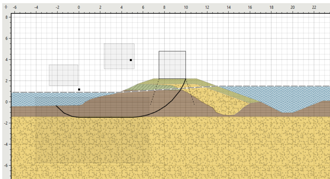
Figuur B2.1.4: Dijkvak 10 VO, STBI, variant met versterking in grond (klei) met een verkeersbelasting van 13 \text{ kN/m}^2 . Berekende SF = 1,01 .
