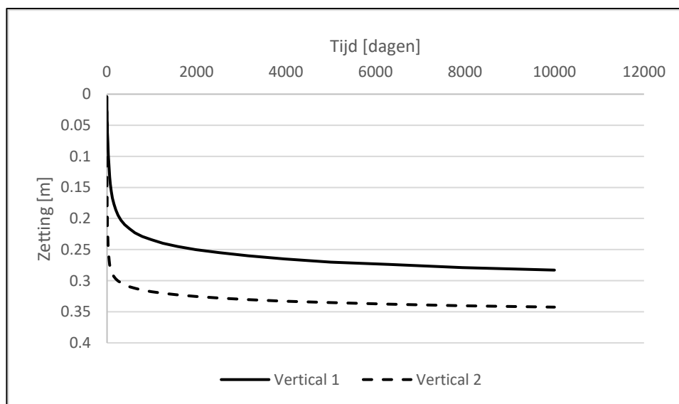
Figuur 9B.2: dijkvak 9B, berekend zettingsverloop op twee locaties van de kruin.
