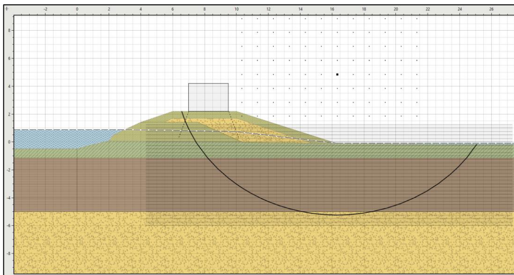
Figuur B2.2.6: Dijkvak 11A SO, STBU variant met versterking in grond (klei). Berekende SF = 1,44.
