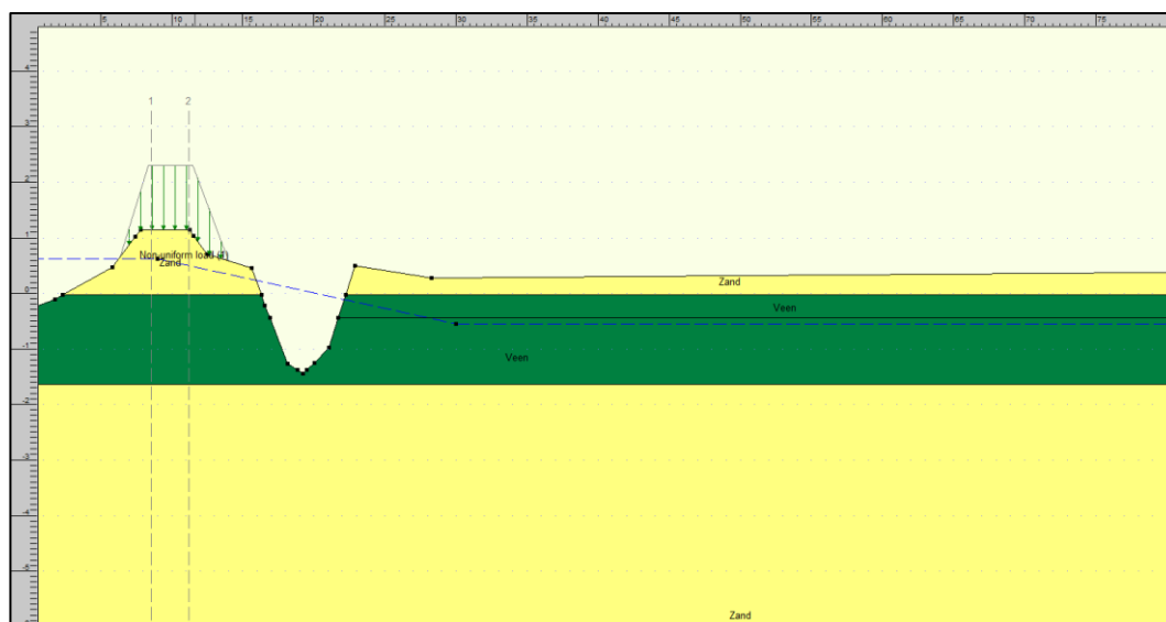
Figuur 9AB.1: Dijkvak 9B, schematisatie zettingsberekening situatie 2004, bodemopbouw conform HA_7.
