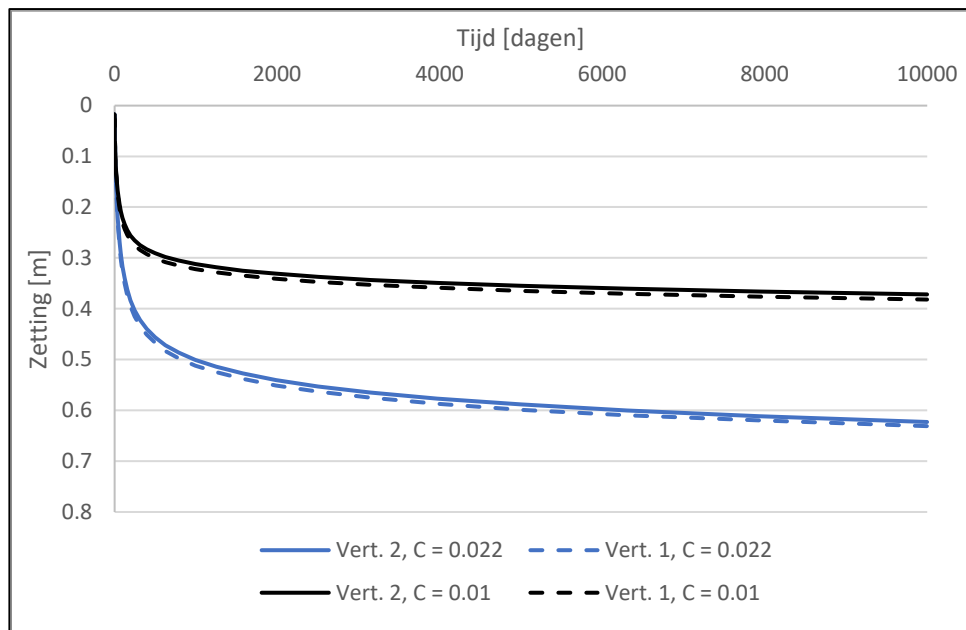
Figuur 9AA.2: Dijkvak 9A, berekende zettingen dijkversterking situatie 2004.
