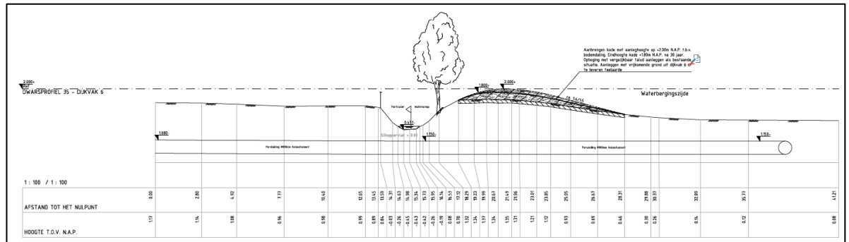
Figuur 7-3: VO Dwarsprofiel van voorgenomen versterking.
