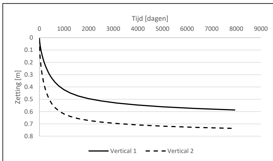
Figuur 12.2: dijkvak 12, berekend zettingsverloop op twee locaties van de kruin.
