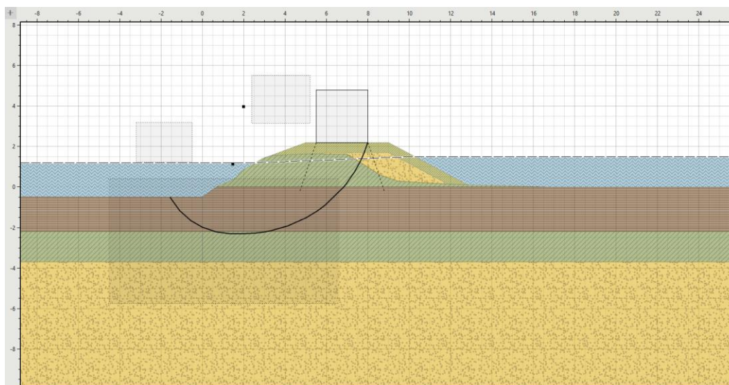
Figuur B2.1.6: Dijkvak 12, STBI, variant met versterking in grond (klei), Zonder opbarsten ter plaatse van binnenzijde meegenomen met een verkeersbelasting van 13 \text{ kN/m}^2 . Berekende SF = 1,15 .
