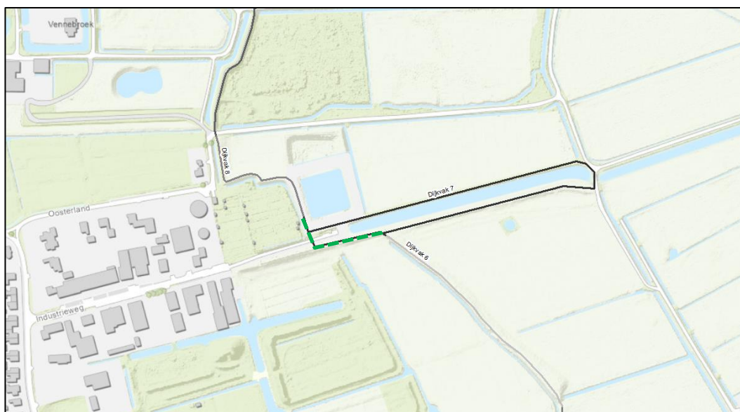
Figuur 9-1: Overzichtstekening dijkvak 8 met het trajectdeel van dijkvak 7 (gestippeld in groen).
