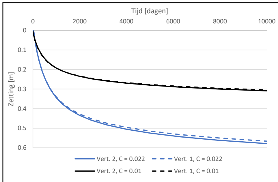
Figuur 13A.2: Dijkvak 13, berekende zettingen dijkversterking situatie 2013.
