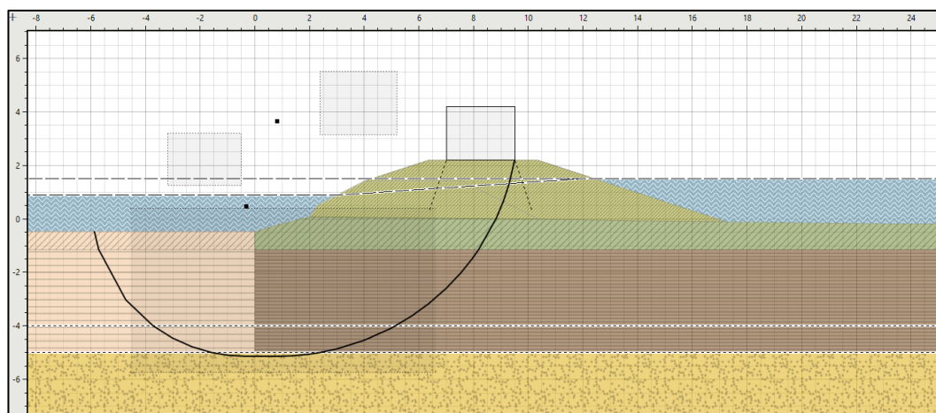
Figuur B2.1.5: Dijkvak 11A SO; opbarsten, STBI, variant met versterking in grond (klei), opbarsten ter plaatse van binnenzijde meegenomen. Berekende SF = 0,90.
