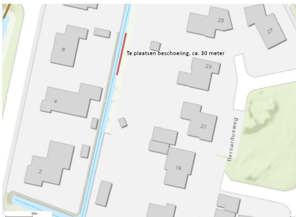
Figuur 1: Locatie van werkzaamheden. De rode lijn geeft de aan te leggen beschoeiing weer.
