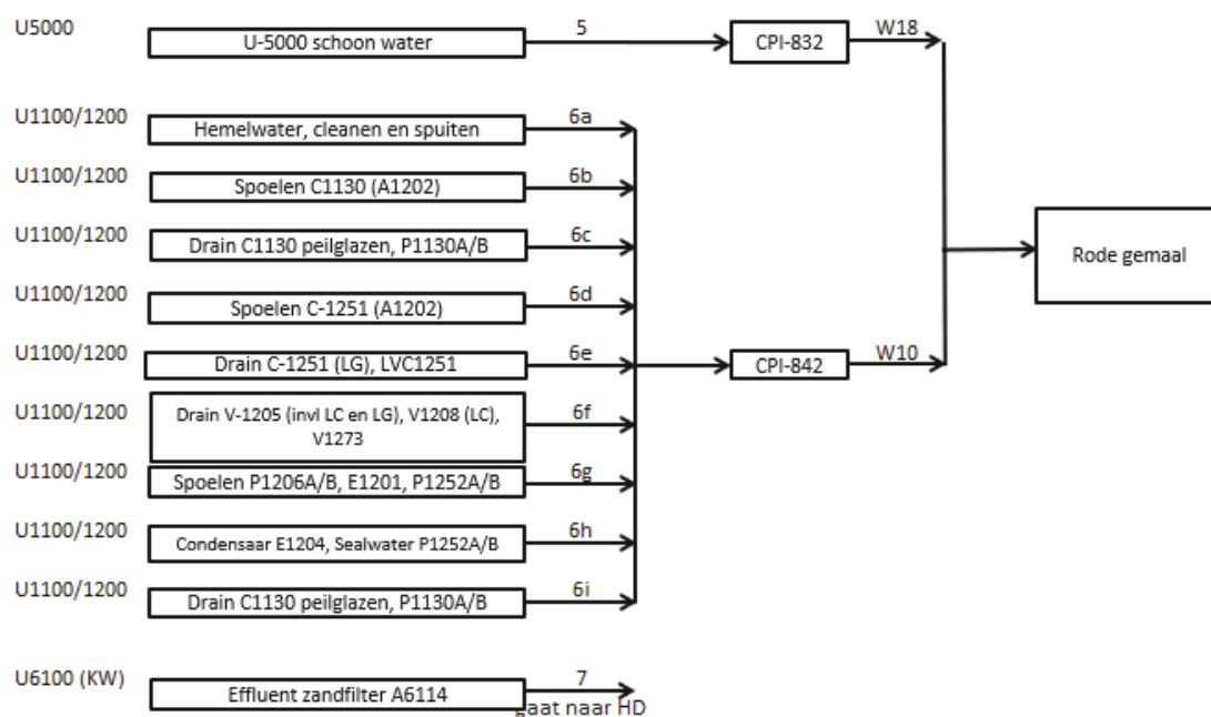
Figuur 6.9: schema waterstromen MSPO 2 deel 2
