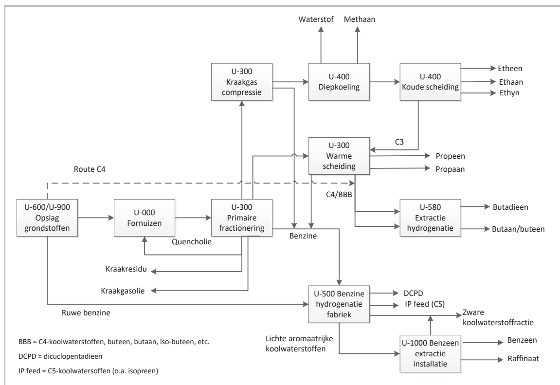
Figuur 4.2 : Prinscipeschema MLO
