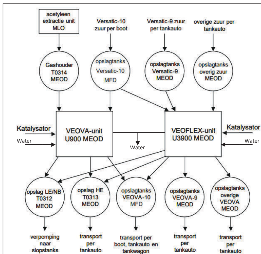
Figuur 4.5: Overzicht MVEO Veova/Veovaflex
