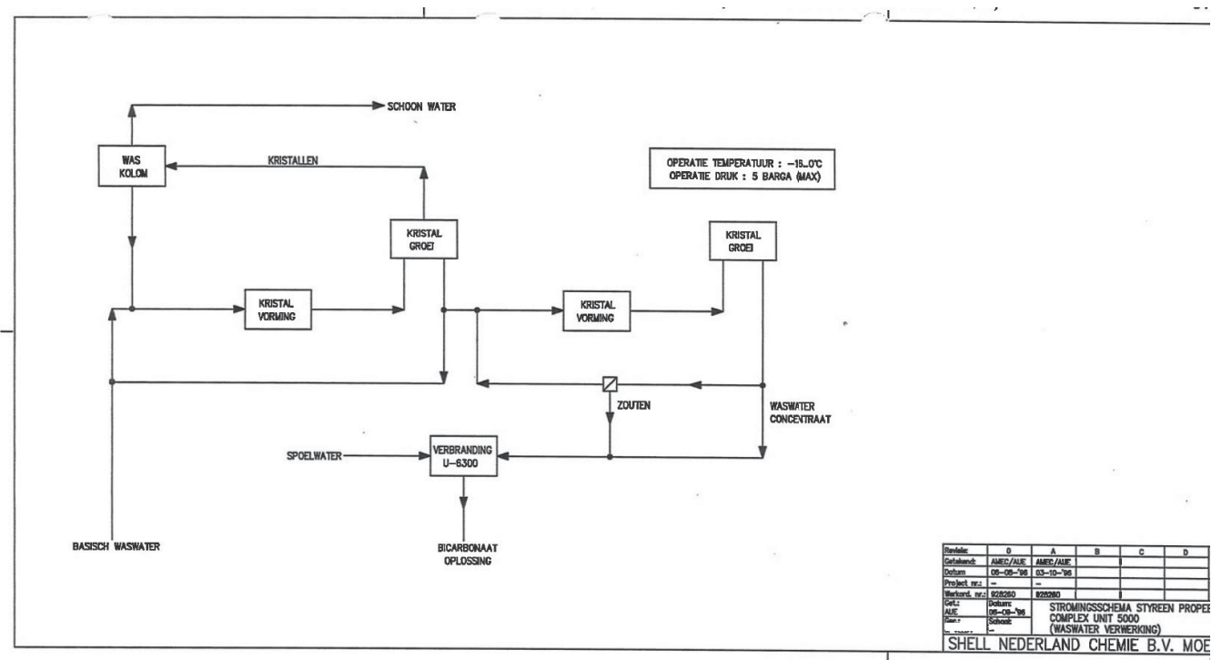
Figuur 1, Gesimplificeerde weergave MSPO2 NIRO unit.
