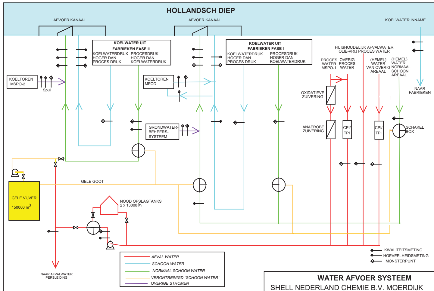
Figuur 6.1: overzicht waterstromen SNC Moerdijk
