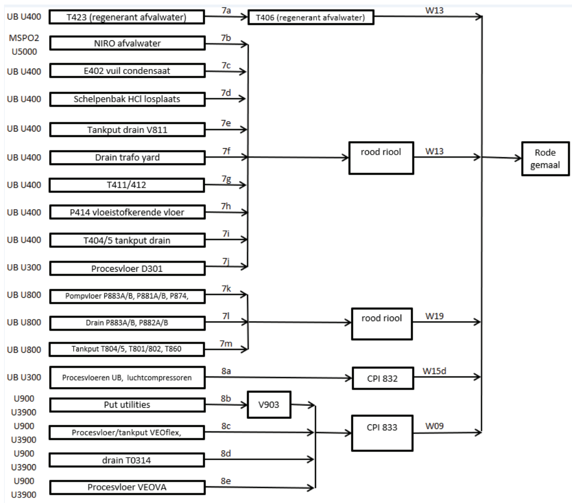
Figuur 6.12: Schema MVEO productie deel 3
