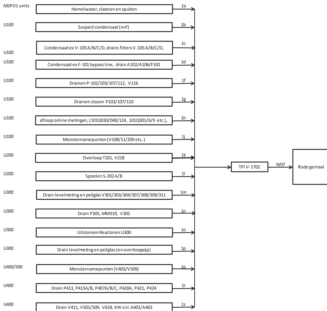
Figuur 6.6 : Waterstromen MSPO 1 deel 1
