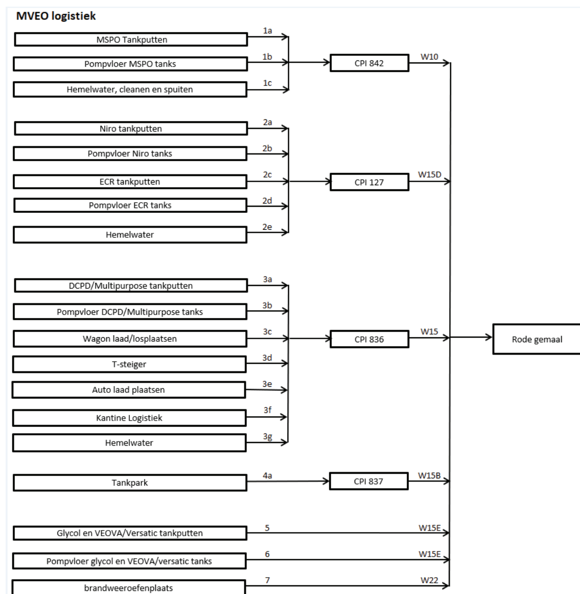
Figuur 6.14: Schema waterstromen MVEO logistiek
