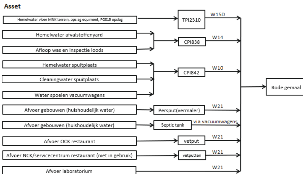
Figuur 6.15 overzicht overige stromen
