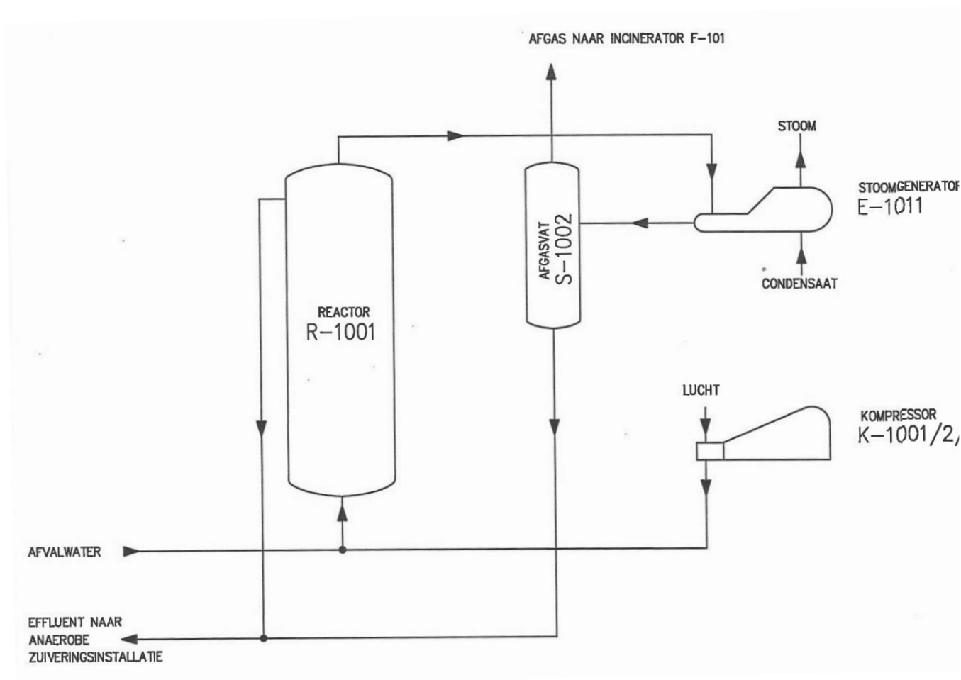
Figuur 1, Gesimplificeerde weergave MSPO1 ZIMPRO unit.
