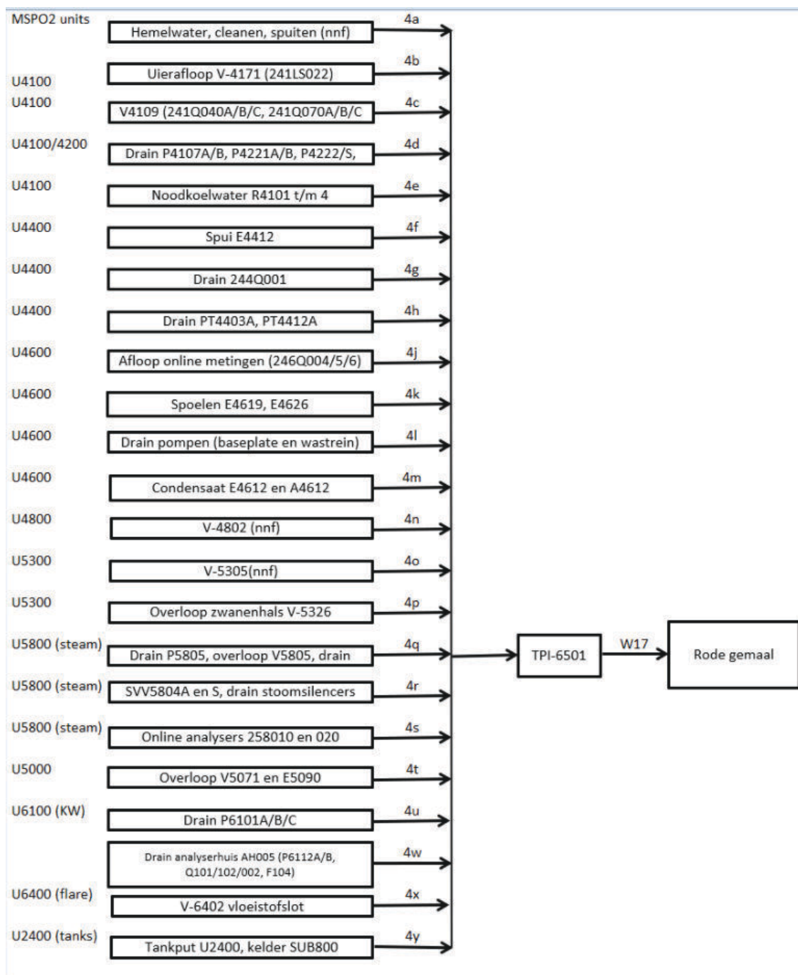
Figuur 6.8: schema waterstromen MSPO2 deel 1
