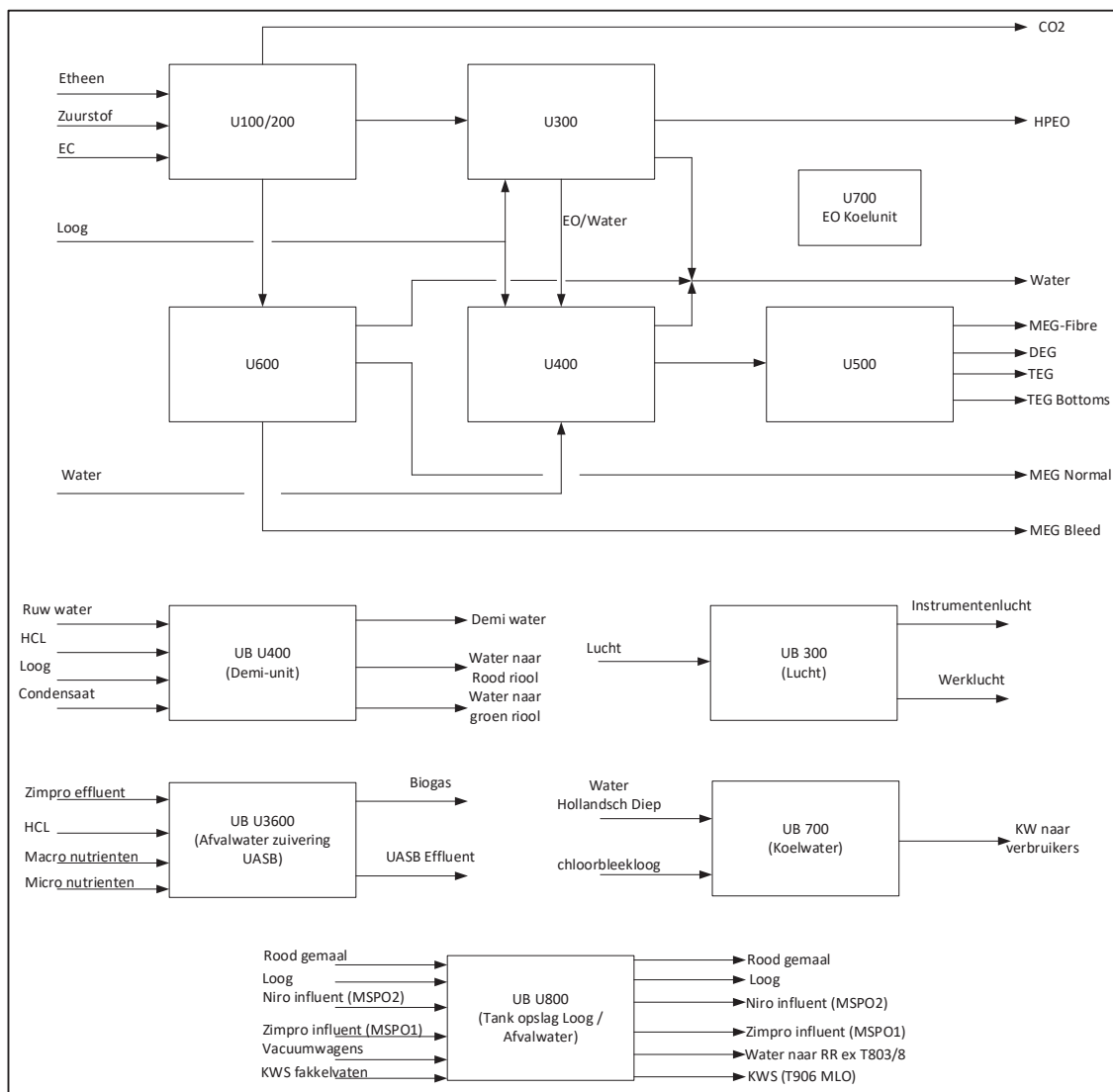
Figuur 4.4: Overzicht MVEO
