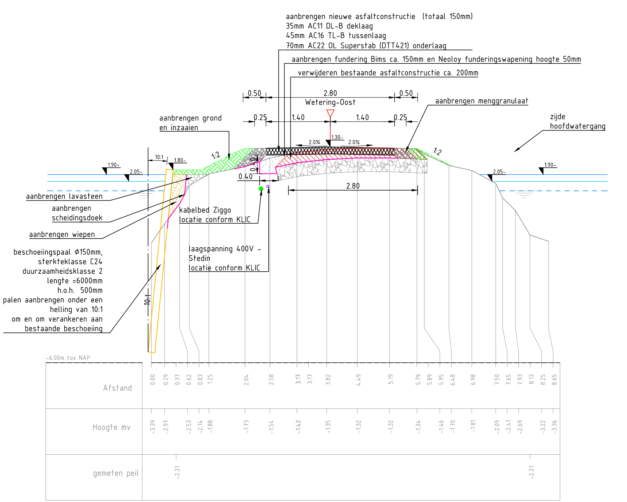
Dwarsprofiel 11-1: wegophoging op Wetering-Oost (lophoging A 0-0,10m) schaal 1:50
