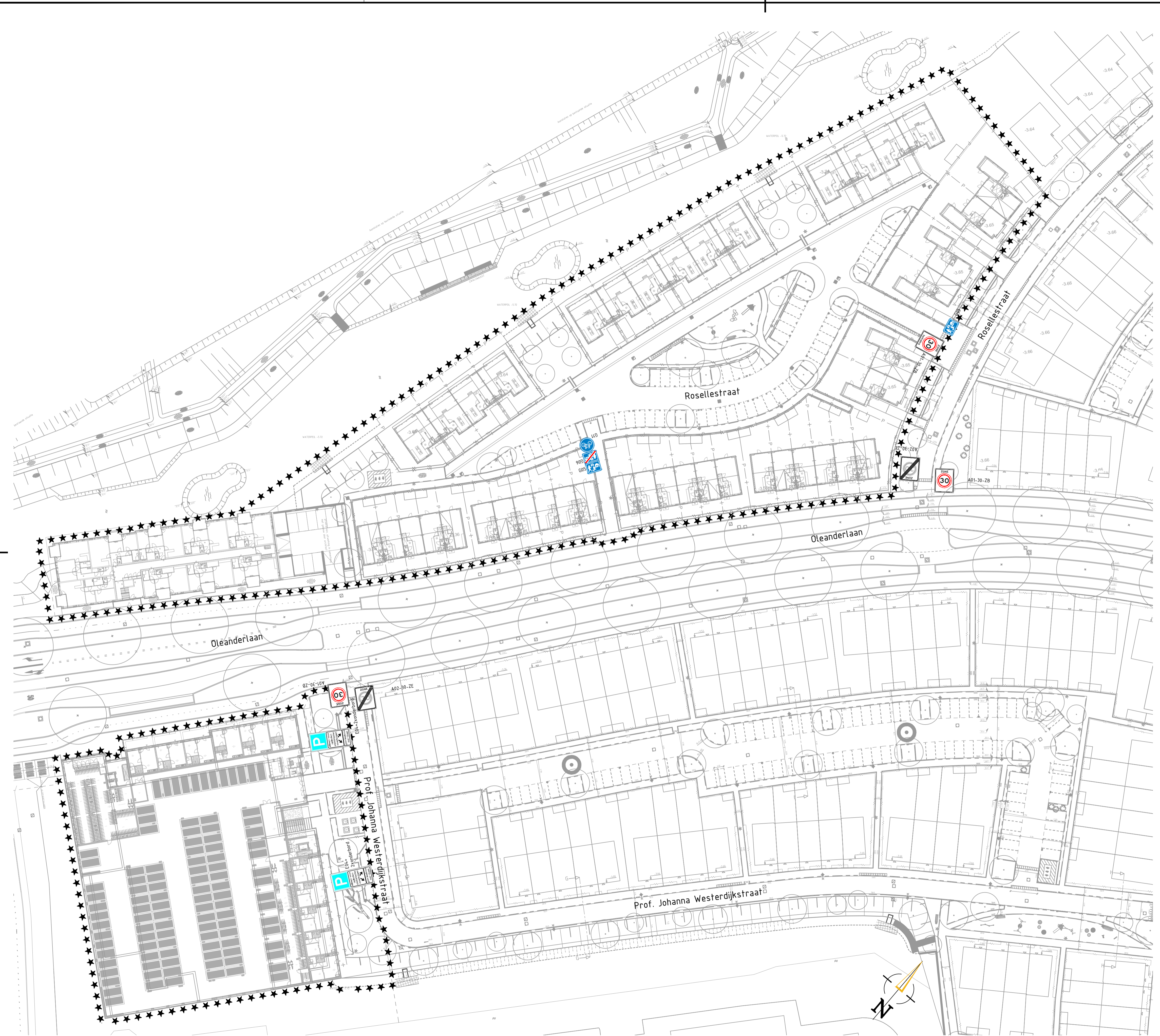
NIEUWE SITUATIE 1 SCHAAL 1:500
