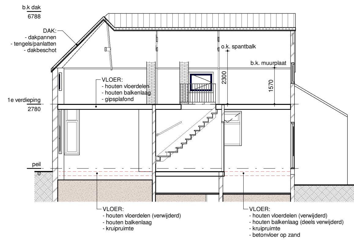
Doorsnede C-C bestand
