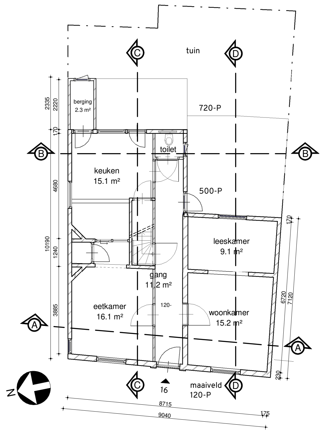
Begane grond - bestand
