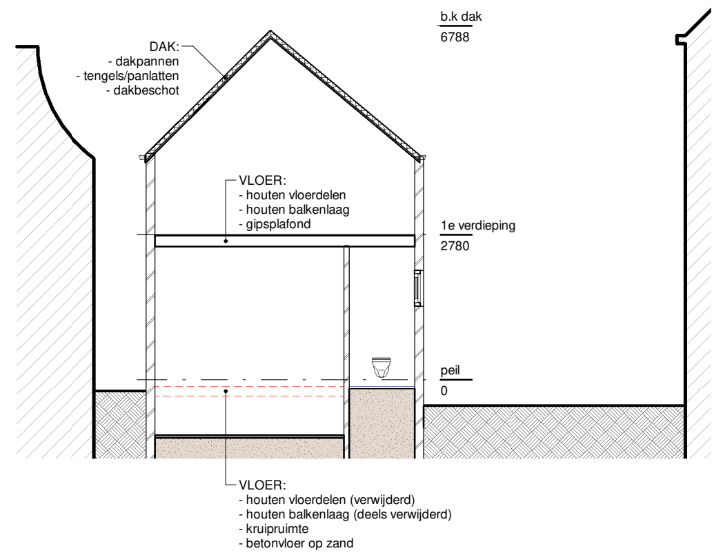
Doorsnede B-B - bestand
