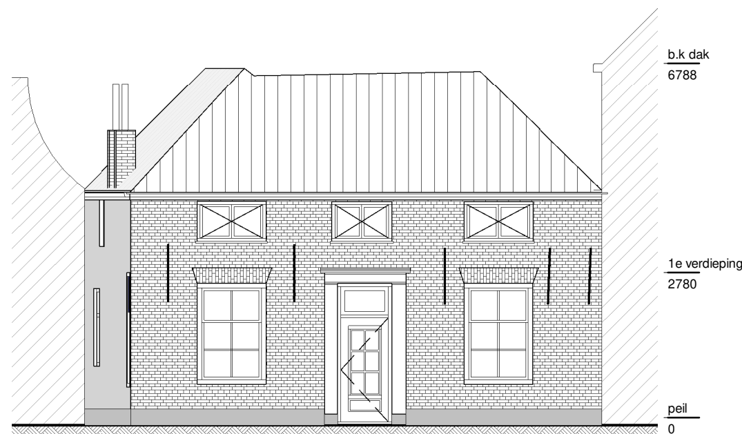
Voorgevel - bestand
