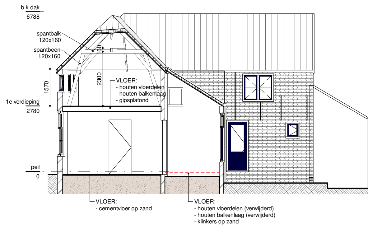
Doorsnede D-D bestand
