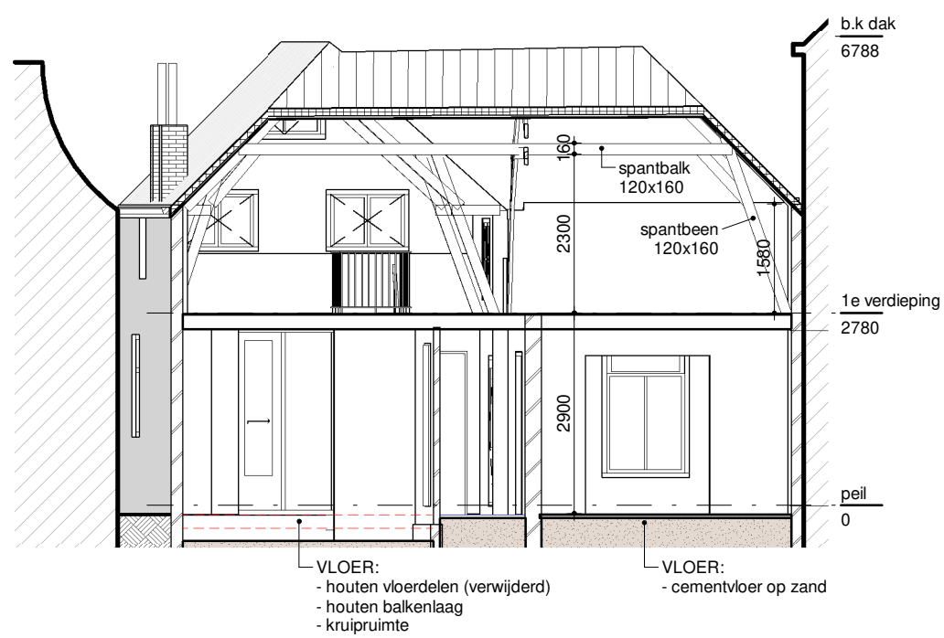
Doorsnede A-A - bestand
