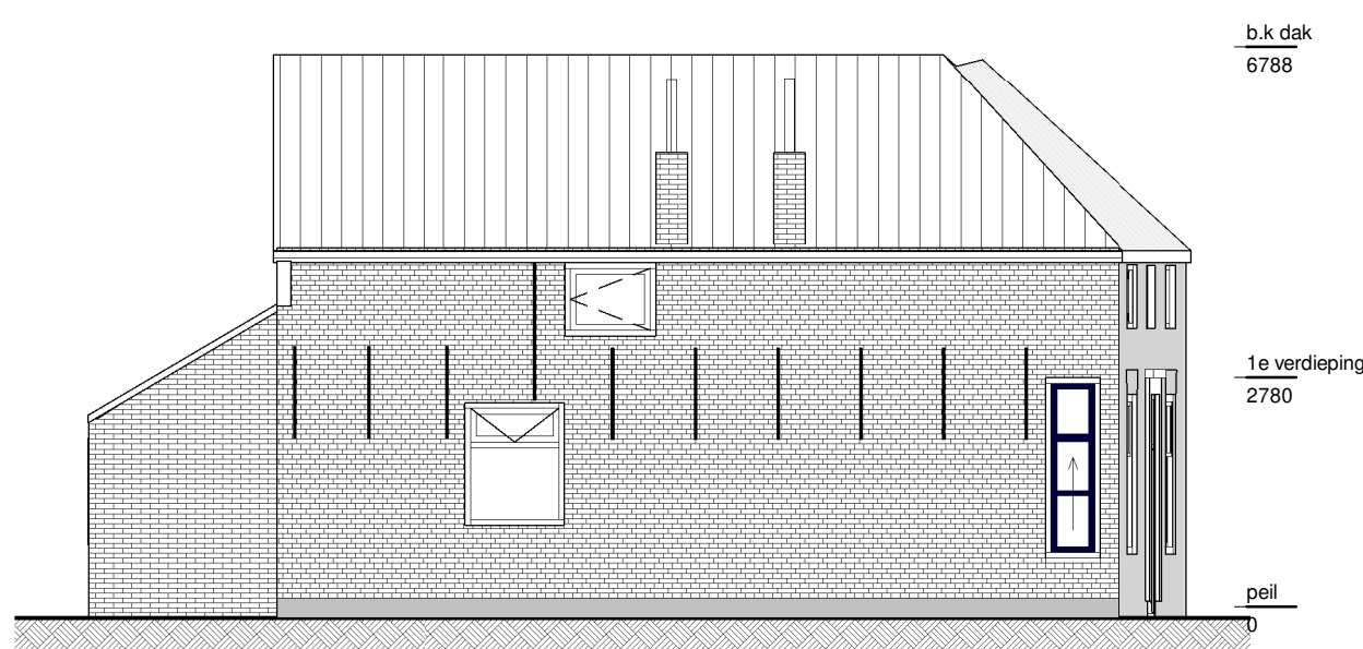
Zijgevel links - bestand
