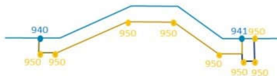
Klei profiel met voor- en achterlandverbetering + Zandontlasting achterland
