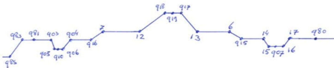
Klei profiel met voor- en achterlandverbetering + Zandontlasting achterland
