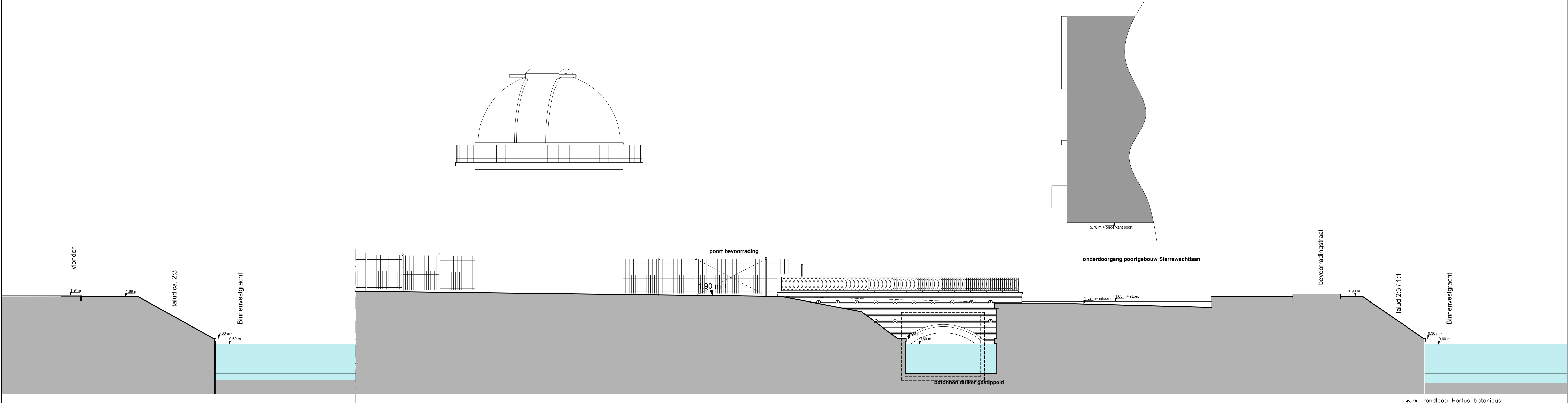
doorsnede A-A
